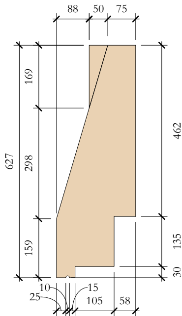
TcS_04 Elevation Right 1 : 10
