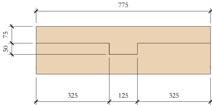
TcS_04 Elevation Top 1 : 10
