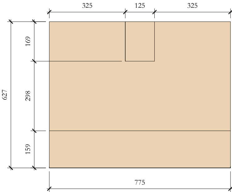
TcS_04 Elevation Front 1 : 10
