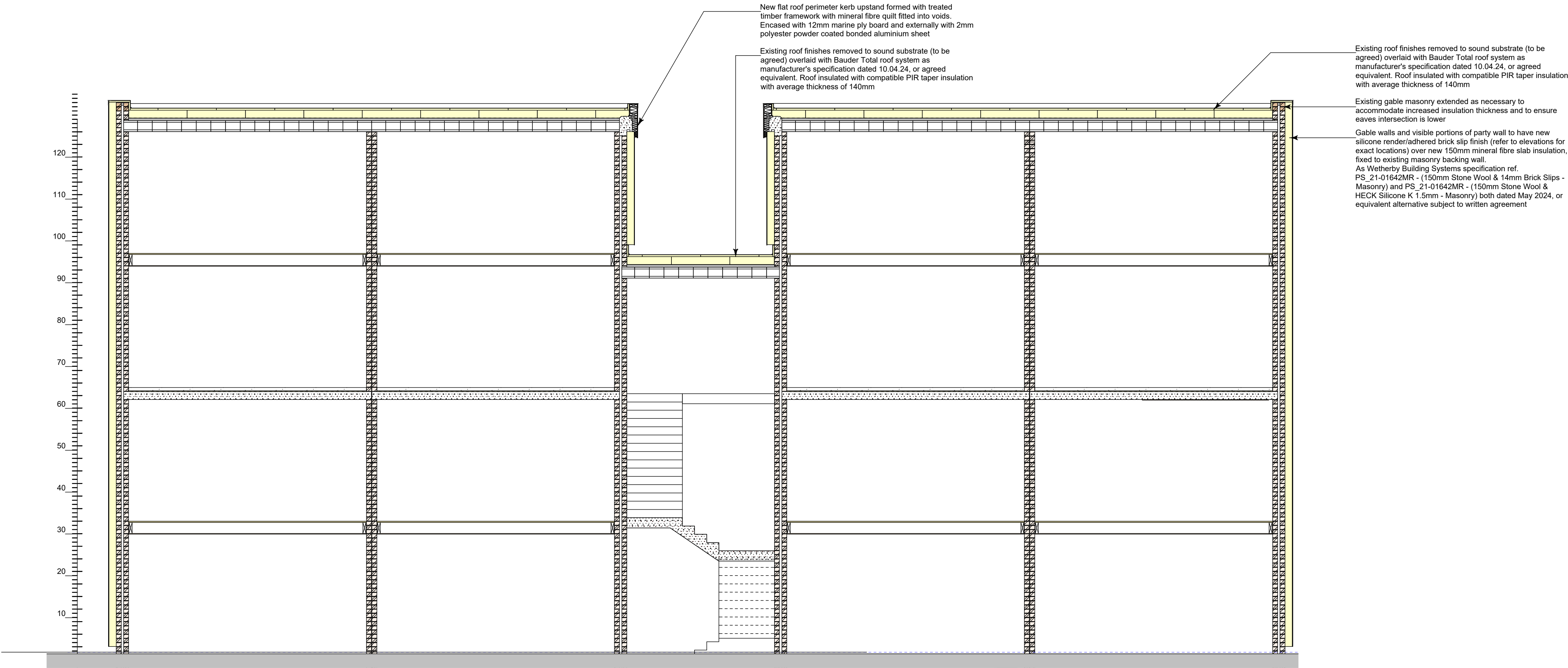
SECTION C-C - MAISONETTE CROSS SECTION (8 UNITS)
