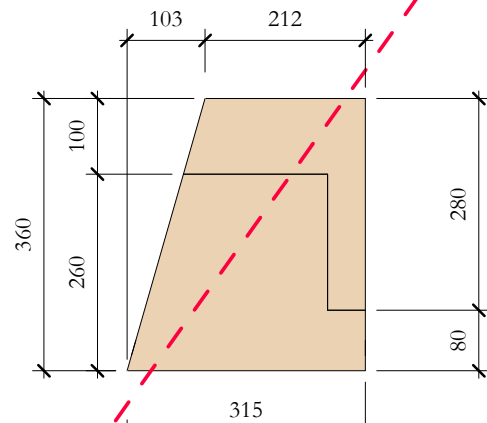
TcP_04 Elevation Top 1 : 10
