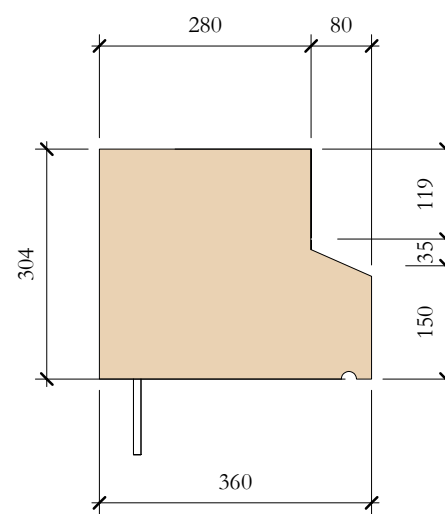
TcP_05 Elevation Left 1 : 10
