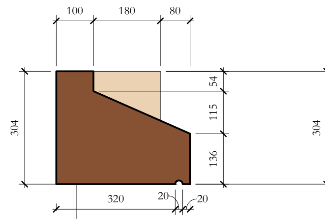
TcP_05 Section AA 1 : 10
