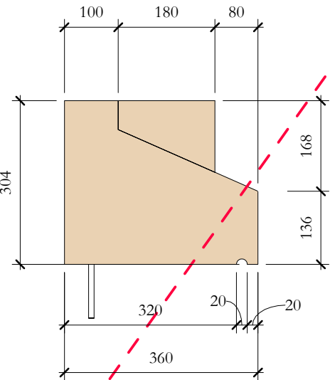
TcP_04 Elevation Left 1 : 10
