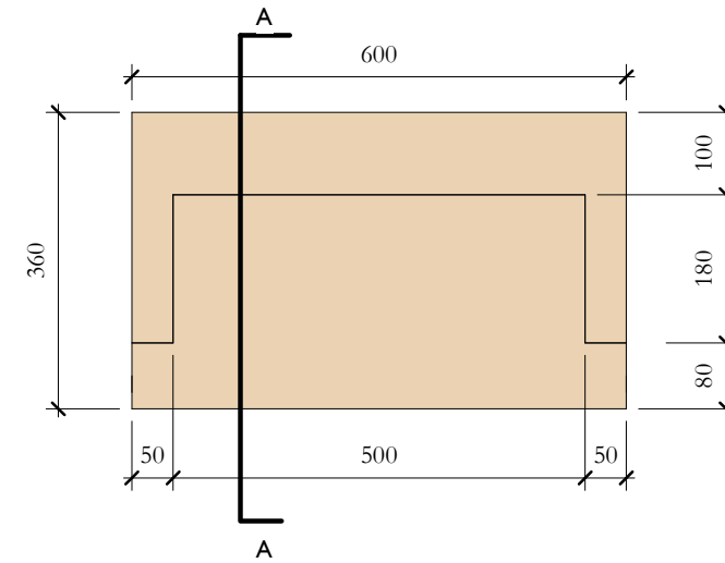
TcP_05 Elevation Top 1 : 10
