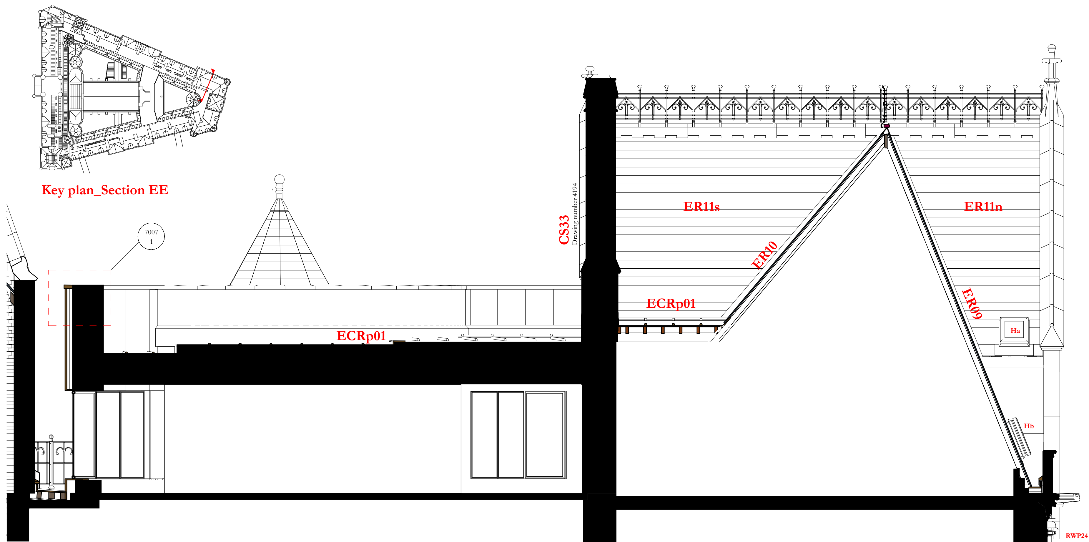
Section EE 1 : 50
