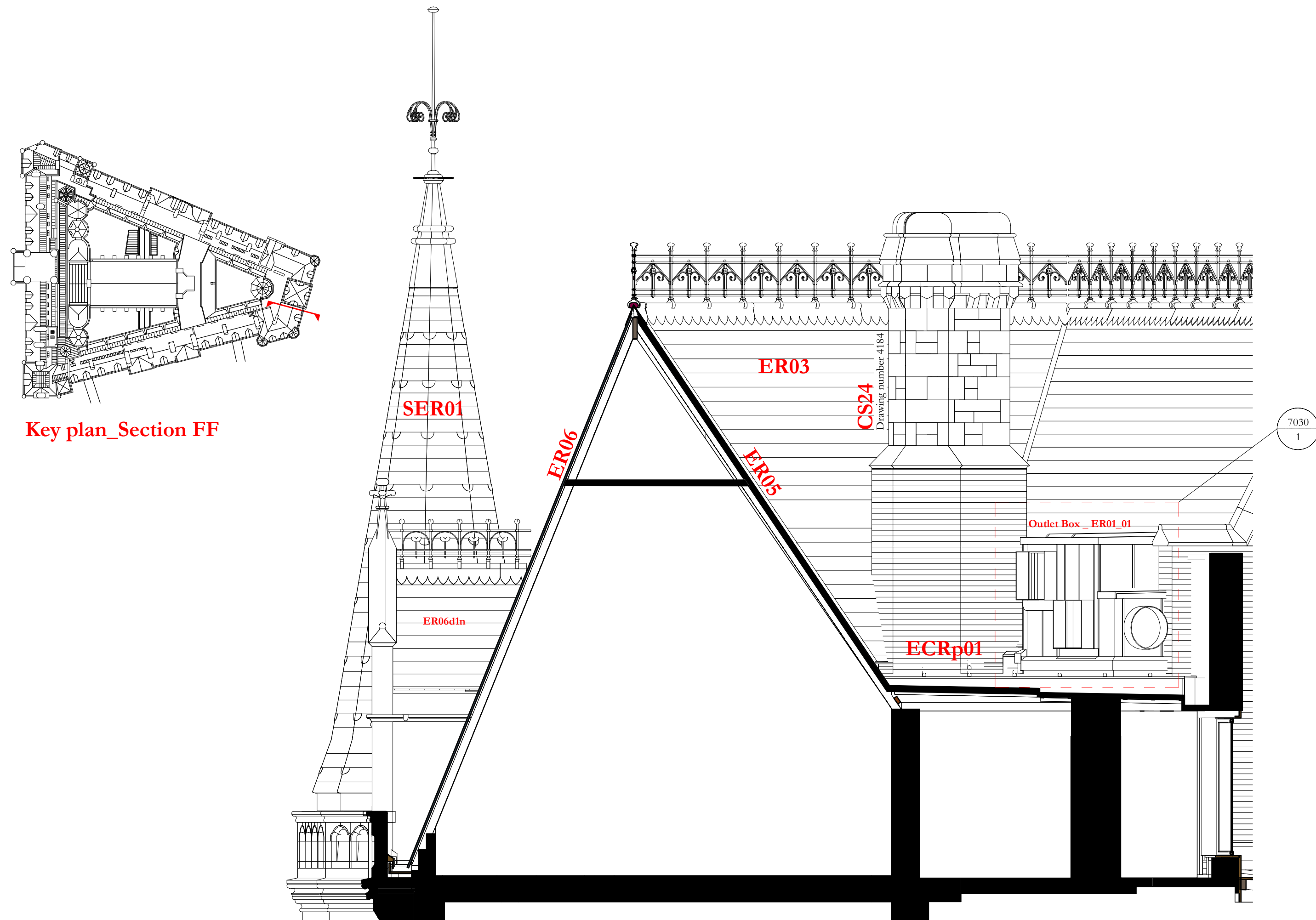
Section FF 1 : 50
