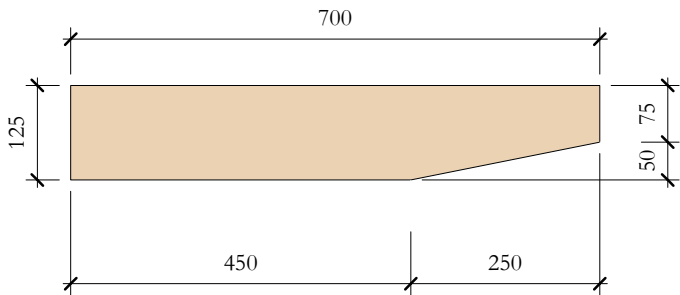
TcW_07 Elevation Top 1 : 10
