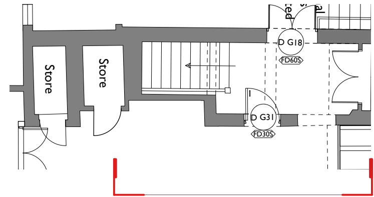
1 Key Plan Scale: 1:100
