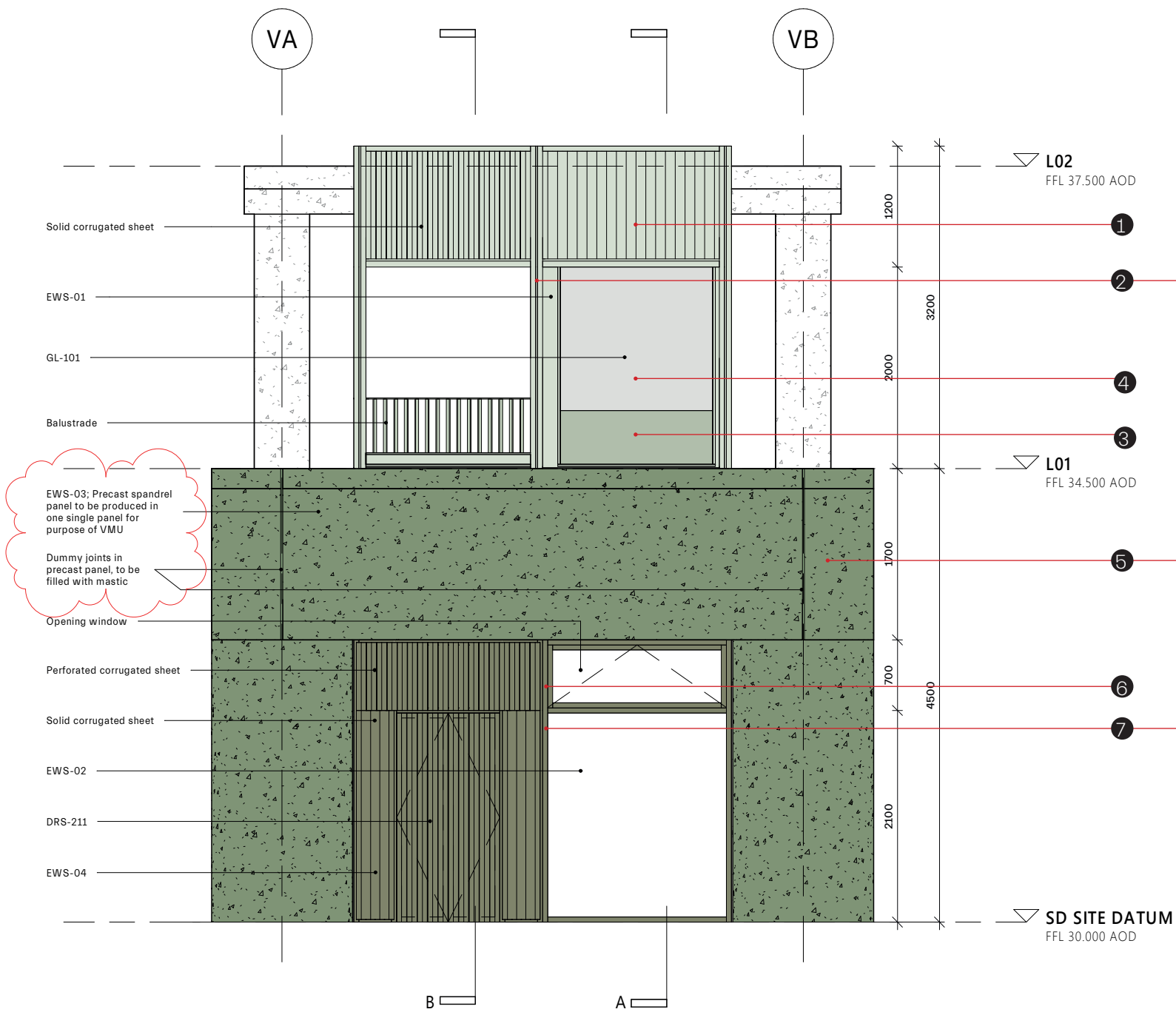
VMU - ELEVATION 1 : 50
