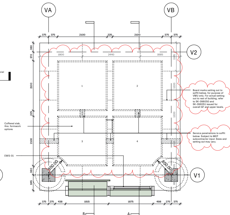
03 VMU - L01 FLOOR PLAN 021481 1:50
