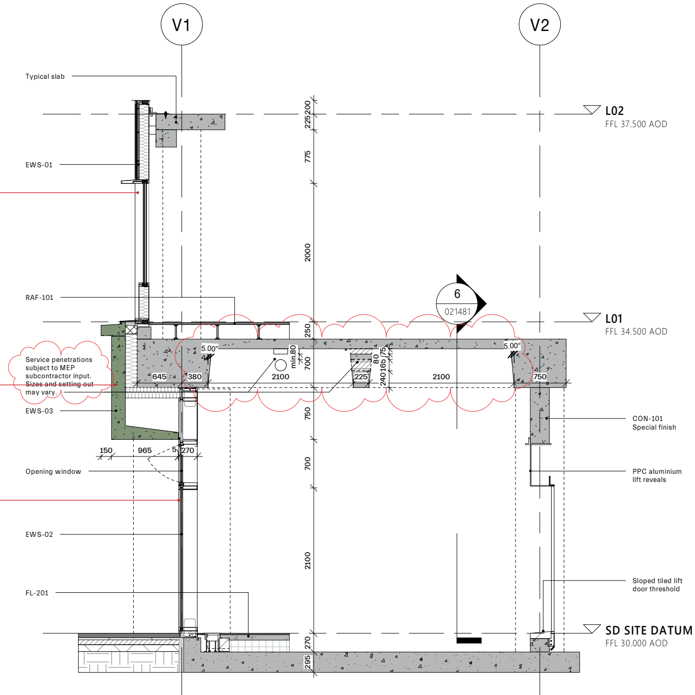
VMU - SECTION A 1 : 50
