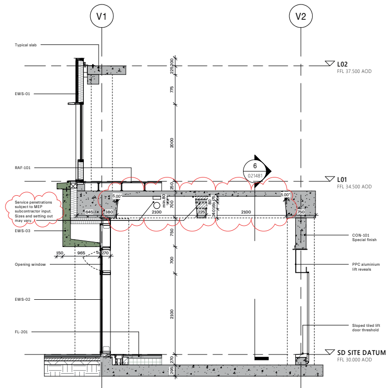
04 VMU - SECTION A 021481 1 : 50
