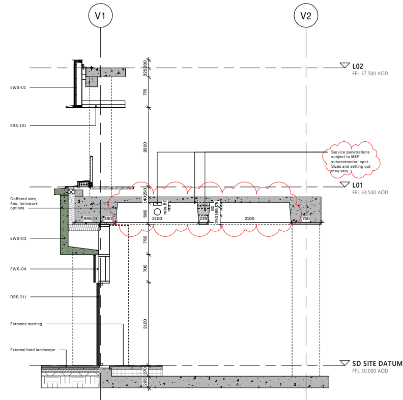
05 VMU - SECTION B 021481 1 : 50
