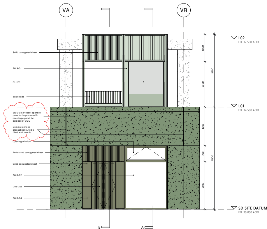
01 VMU - ELEVATION 021481 1:50
