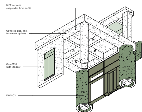
08 VMU - ISO 02 021481)
