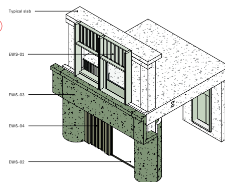
07 VMU - ISO 01 021481
