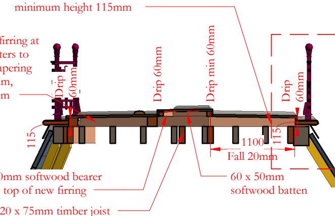
Section D-D
