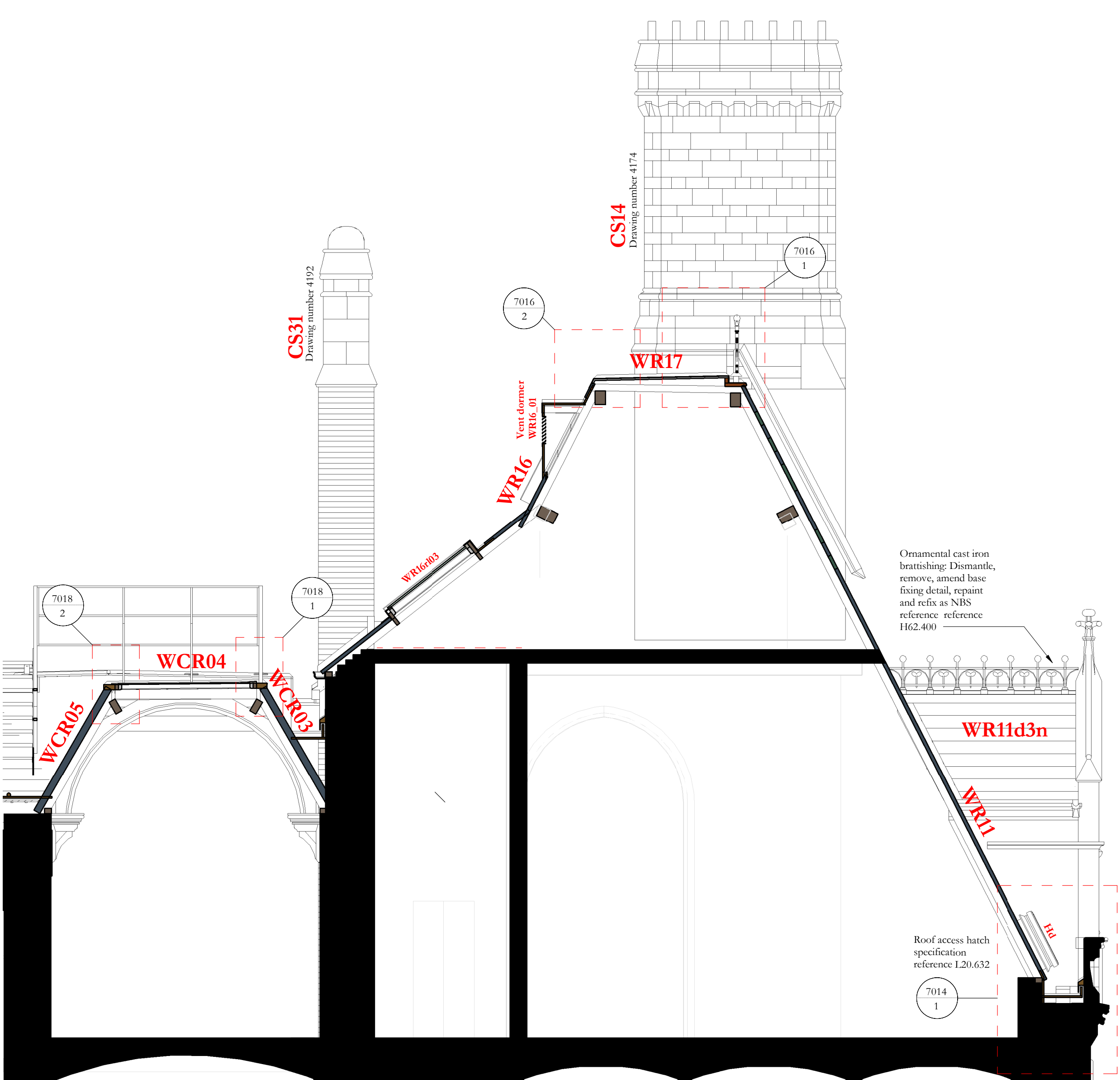
Section WW 1 : 50
