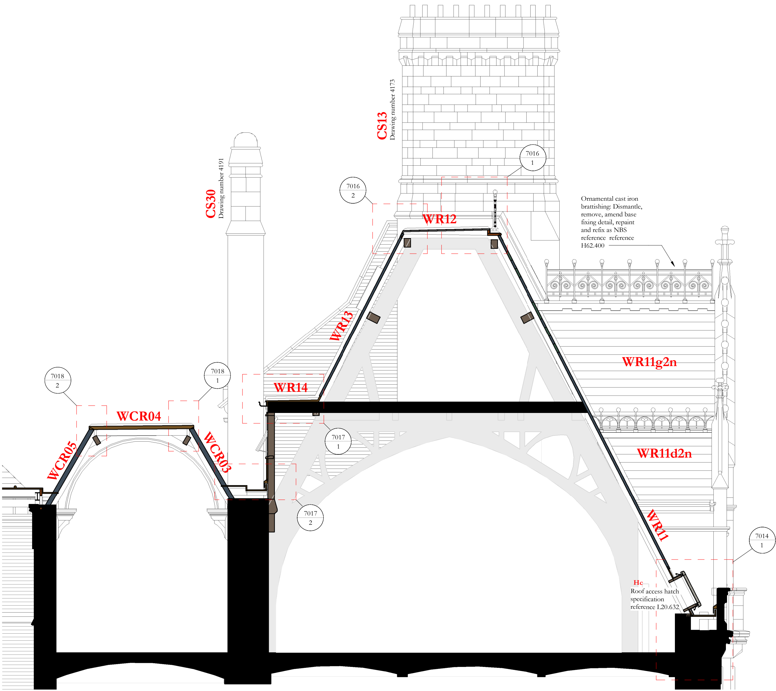
Section VV 1 : 50
