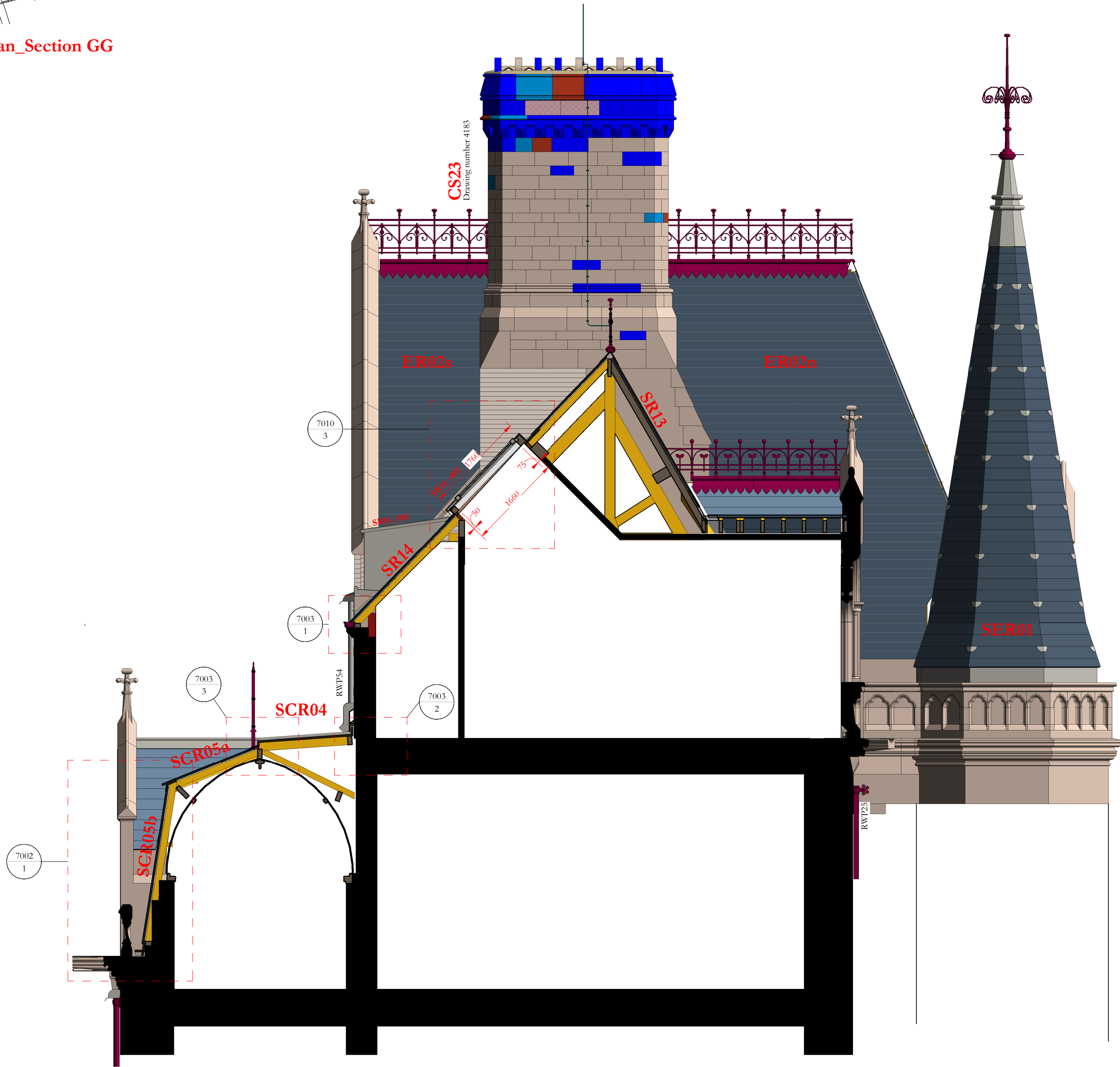
Section GG 1 : 50
