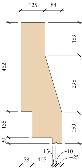
TcS_03 Elevation Left 1 : 10
