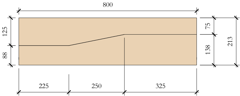
TcS_03 Elevation Top 1 : 10
