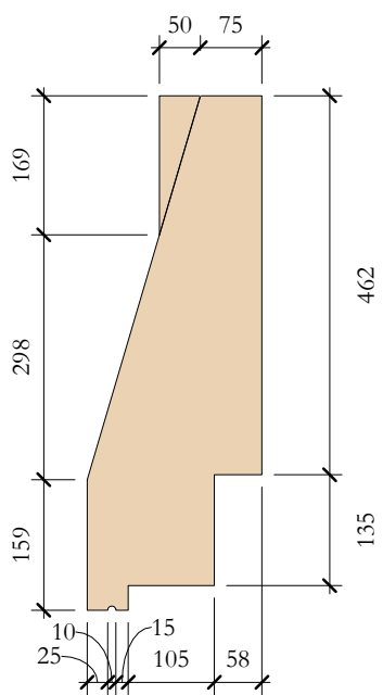
TcS_03 Elevation Right 1 : 10
