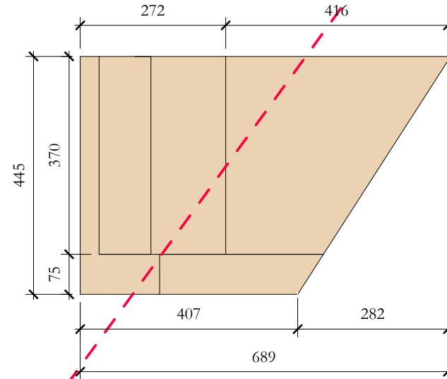
TcA_06 Elevation Top 1 : 10
