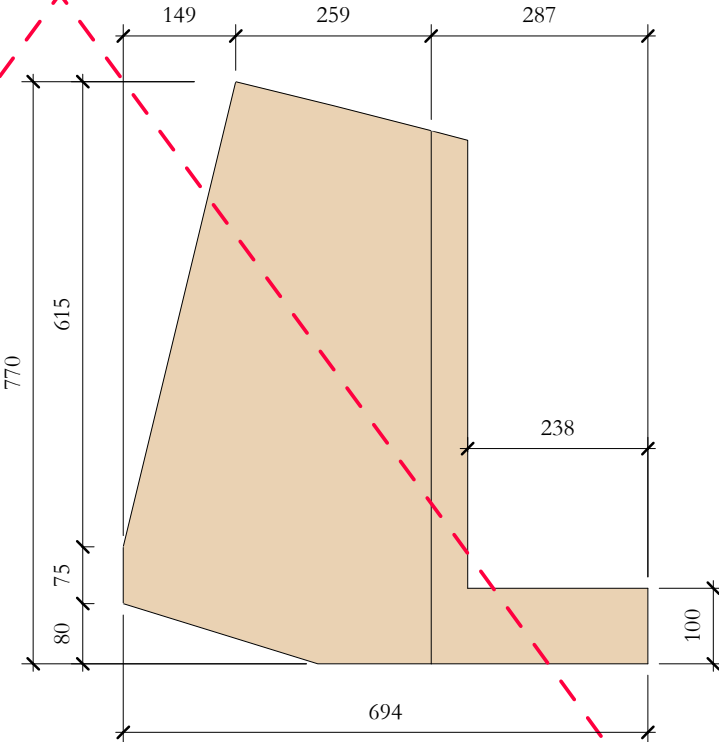
TcA_06 Elevation Front 1 : 10
