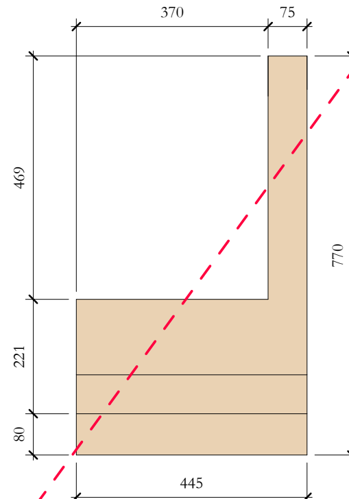
TcA_06 Elevation Left 1 : 10
