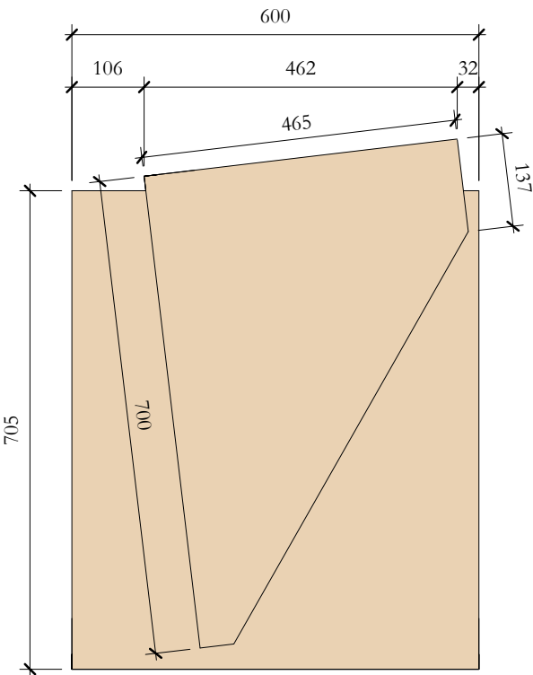
TcC_03 Elevation Top
