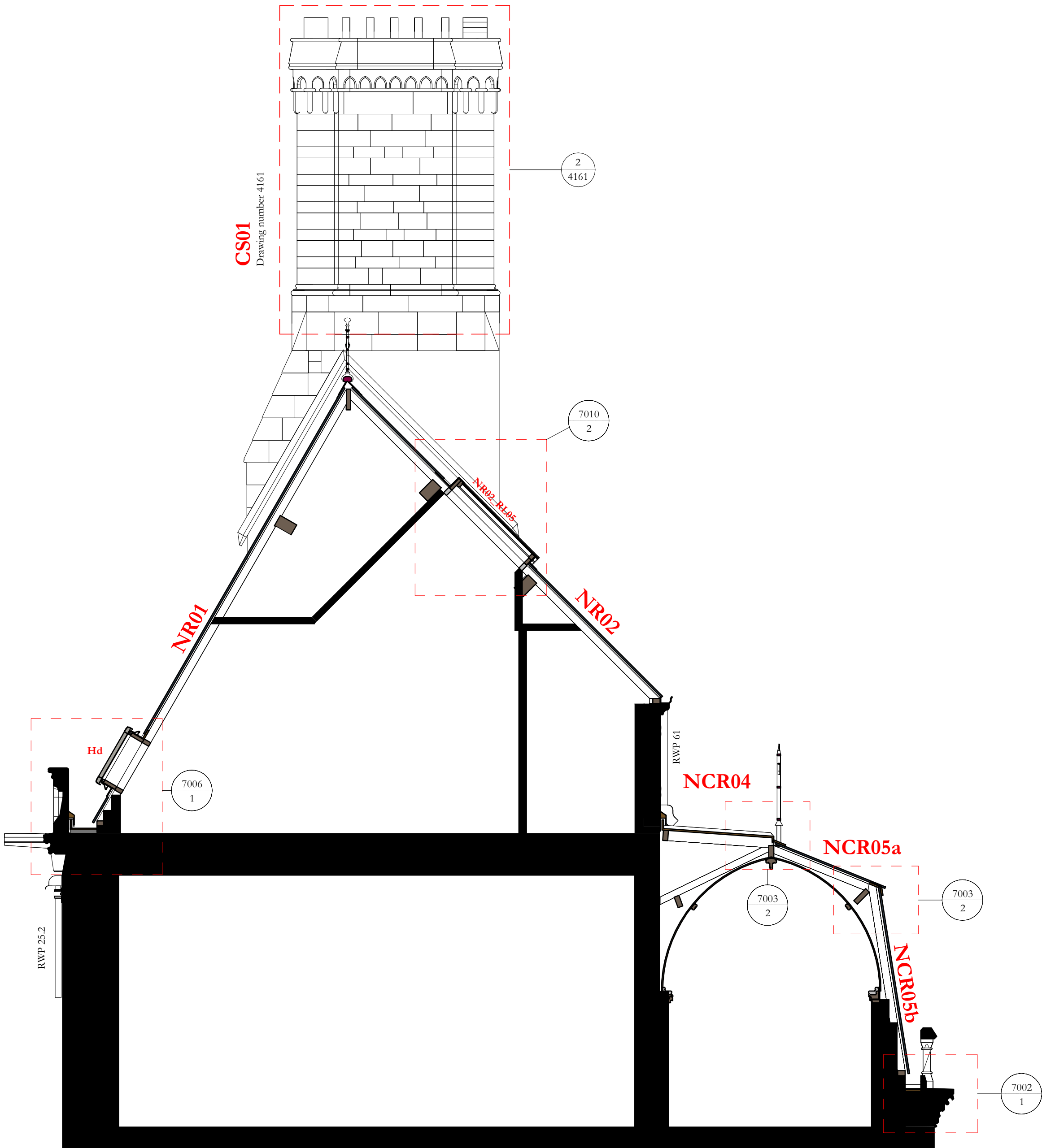
Section CC 1 : 50
