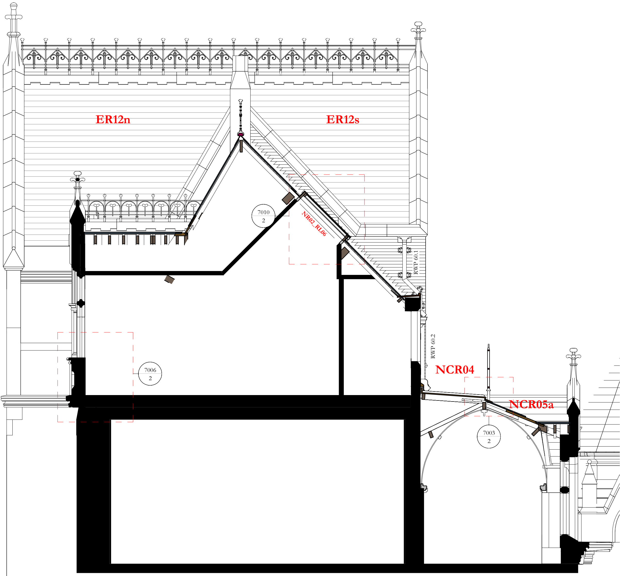
Section DD 1 : 50
