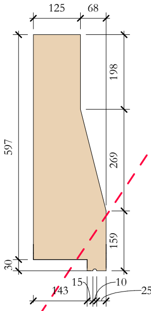
TcS_17 Elevation Left 1 : 10
