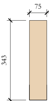
TcR_08 Elevation Left 1 : 10
