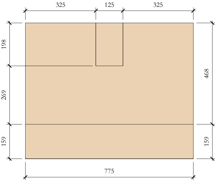
TcS_14 Elevation Top 1 : 10
