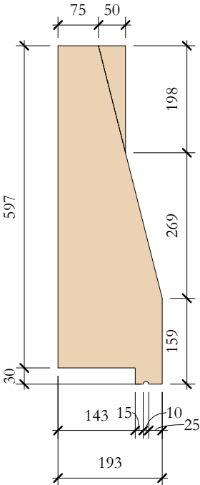
TcS_14 Elevation Left 1 : 10
