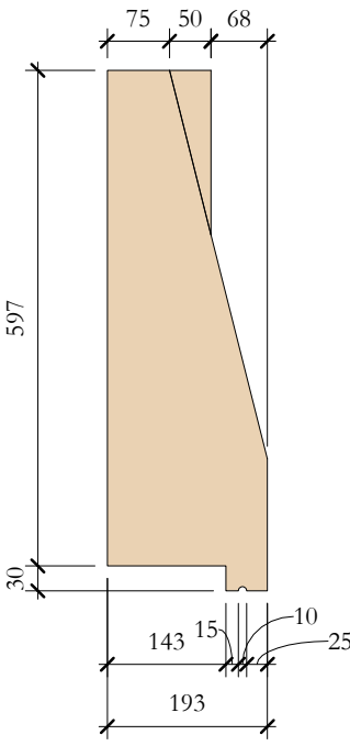
TcS_15 Elevation Left 1 : 10
