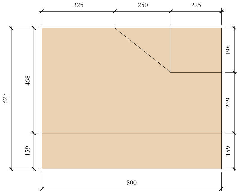
TcS_15 Elevation Top 1 : 10
