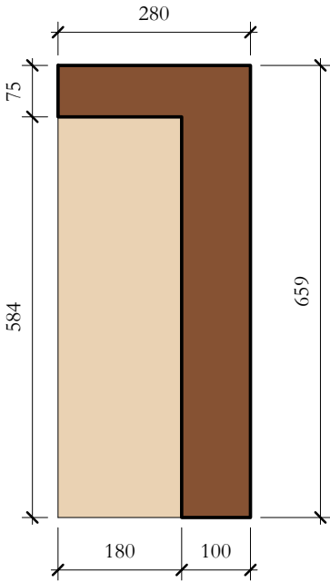
TcP_02 Section AA 1 : 10
