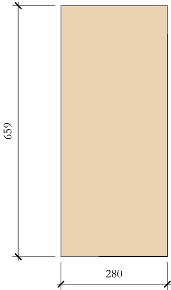
TcP_02 Elevation Left 1 : 10
