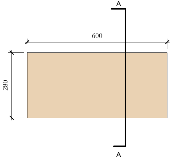
TcP_02 Elevation Top 1 : 10
