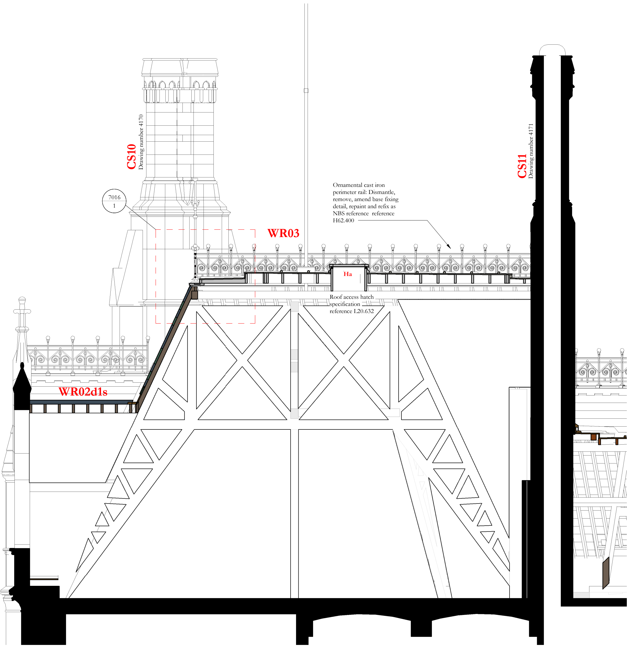
Section RR 1 : 50
