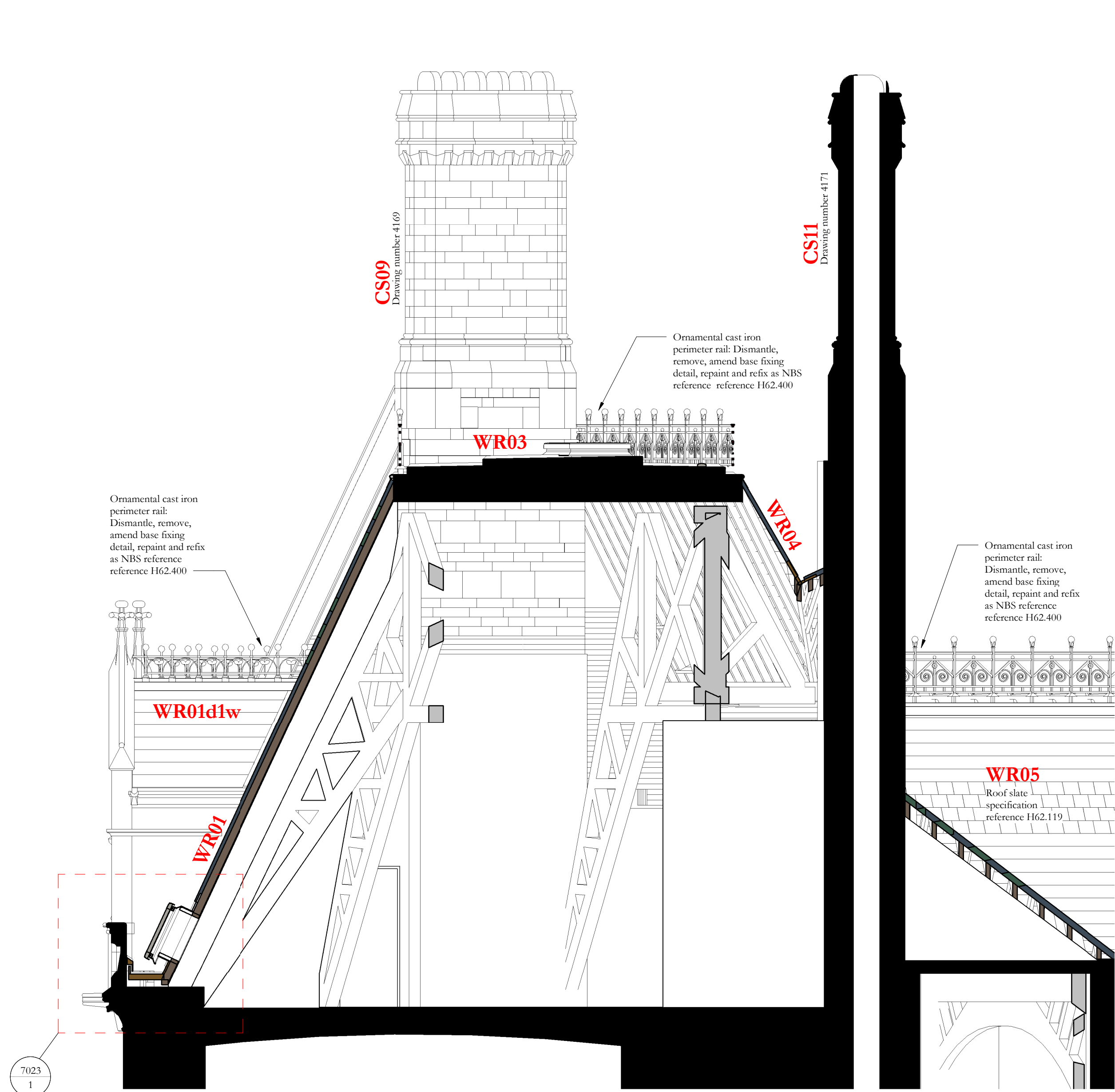
Section QQ 1 : 50
