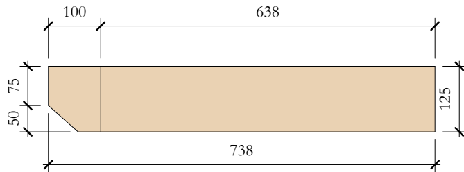
TcV_04 Elevation Top 1 : 10
