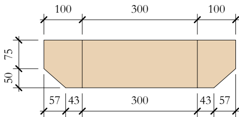
TcV_03 Elevation Top 1 : 10
