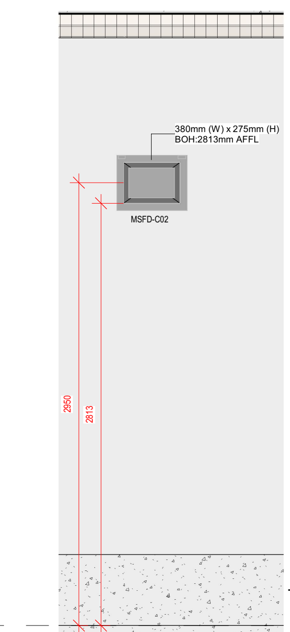
F MSFD-C02 1:25
