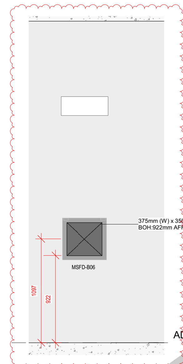
A MSFD-B06 1:25
