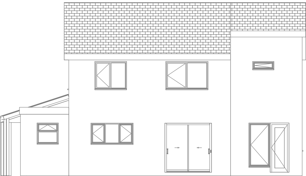
Rear 1 : 100
