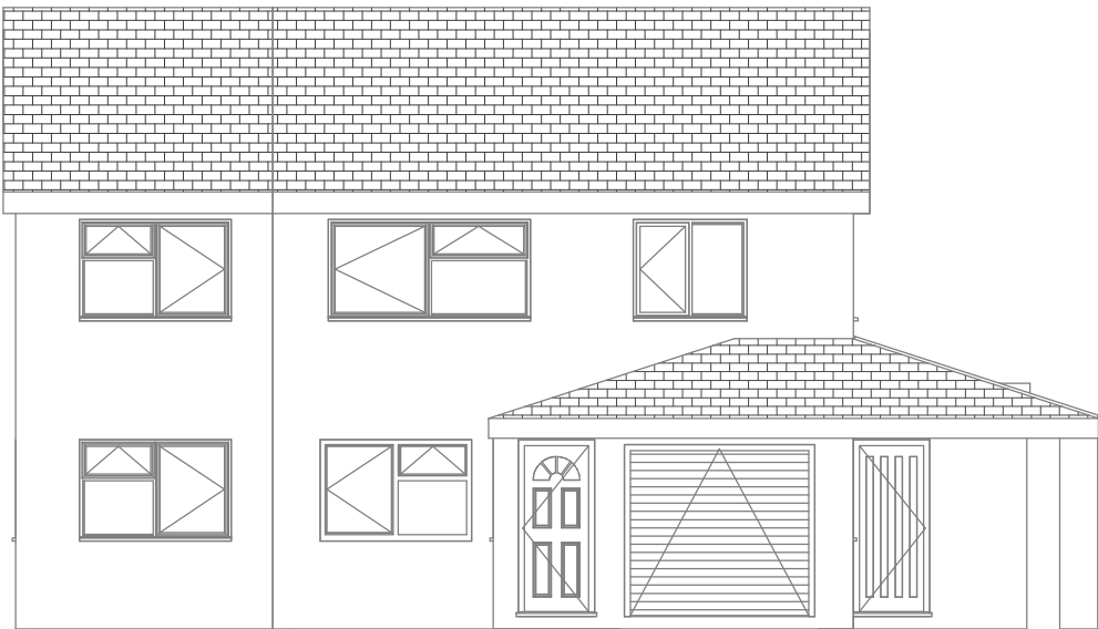
Front 1 : 100
