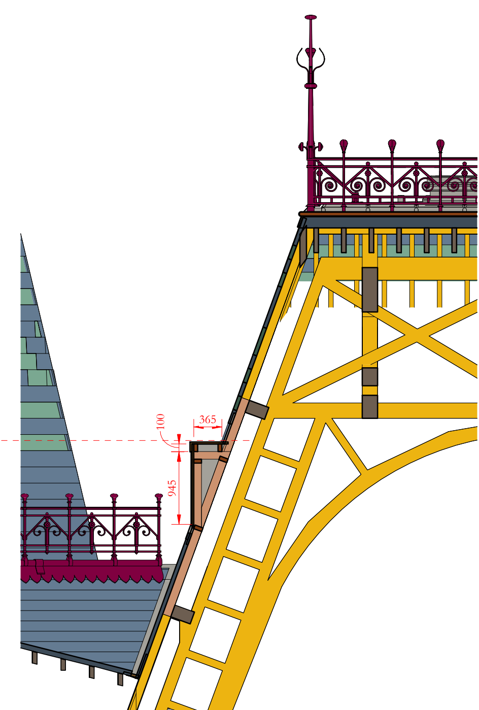
Section A-A
