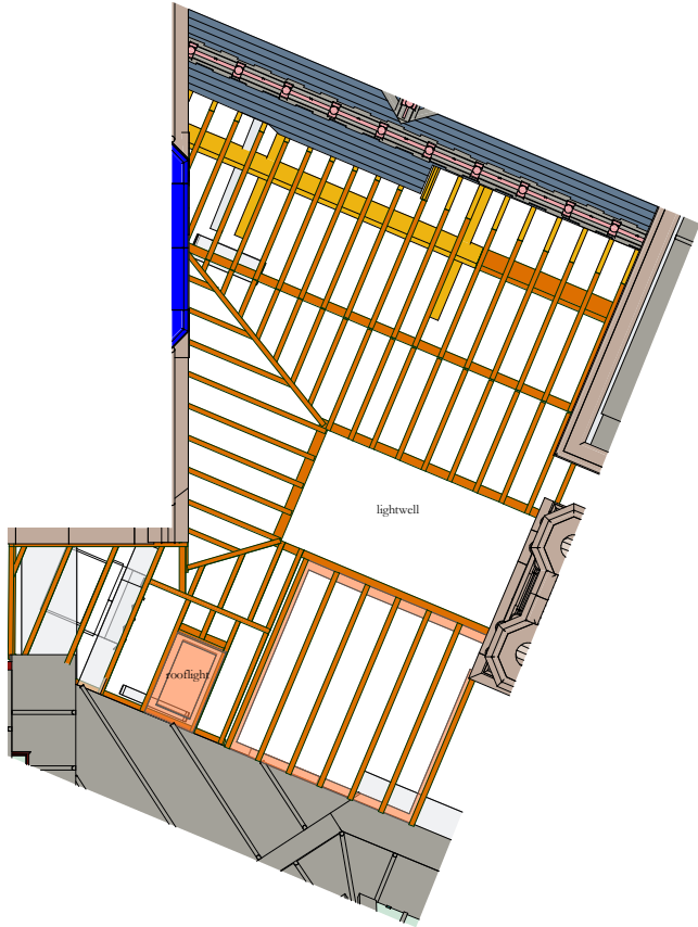
2a Plan Area 2 1 : 50
