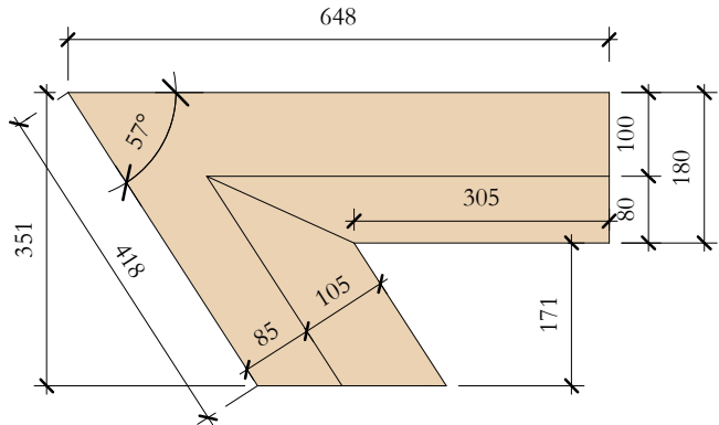
TcP_19 Elevation Top 1 : 10
