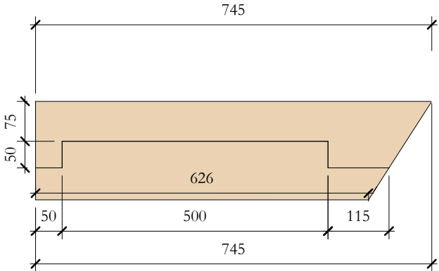
TcP_18 Elevation Top 1 : 10
