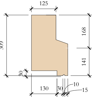
TcP_18 Elevation Left 1 : 10
