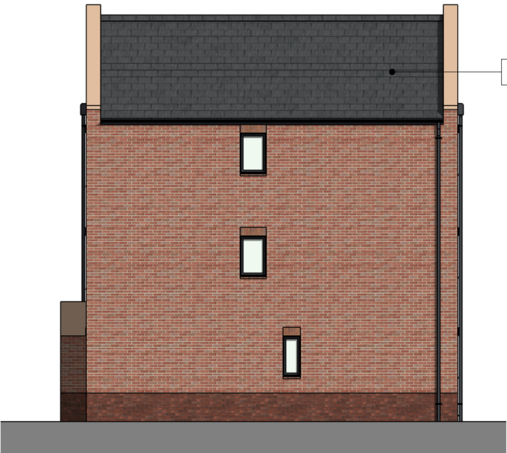
Right Elevation 1 : 100
