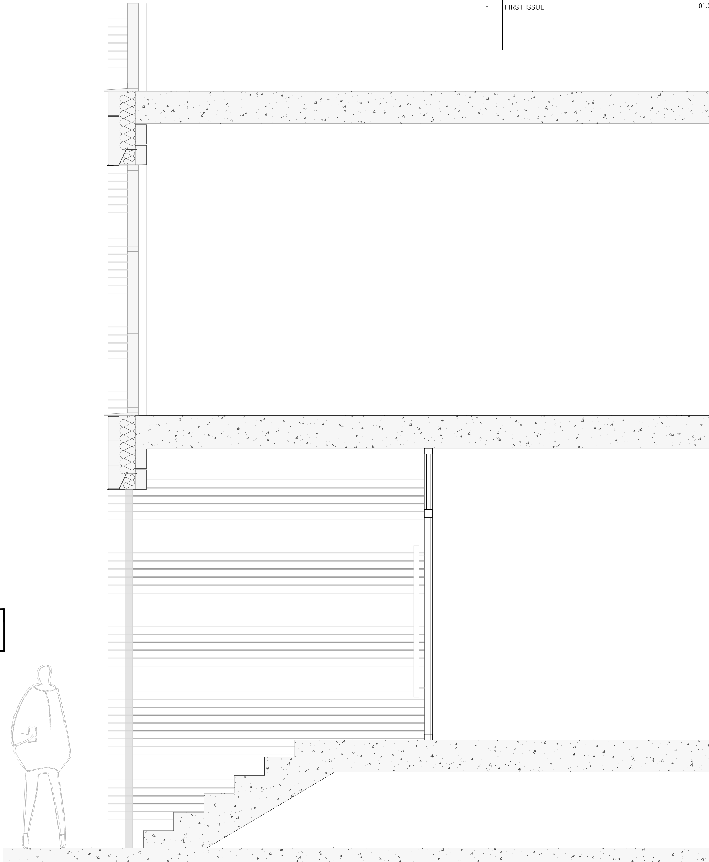
SECTION A:A SCALE 1:20
