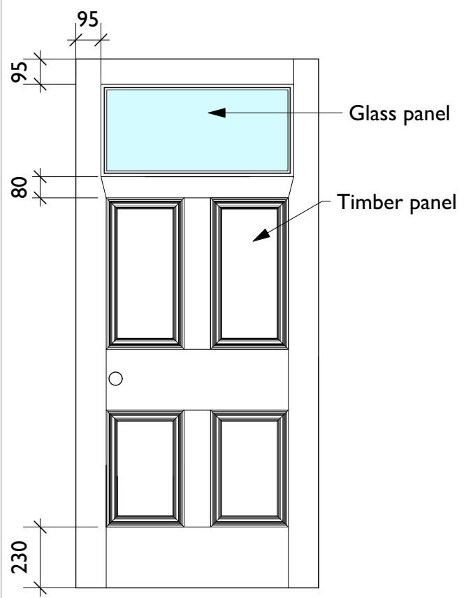
6 Existing Door Type 1 Scale: 1:20
