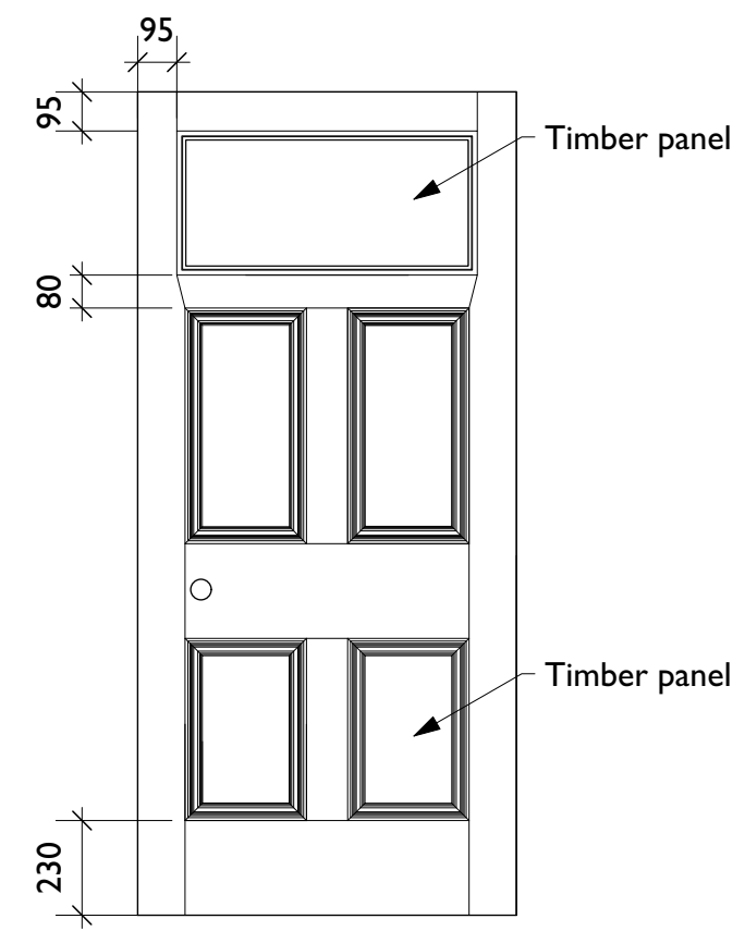
8 Existing Door Type 3 Scale: 1:20
