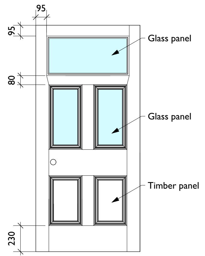
5 Existing Door Type 2 Scale: 1:20
