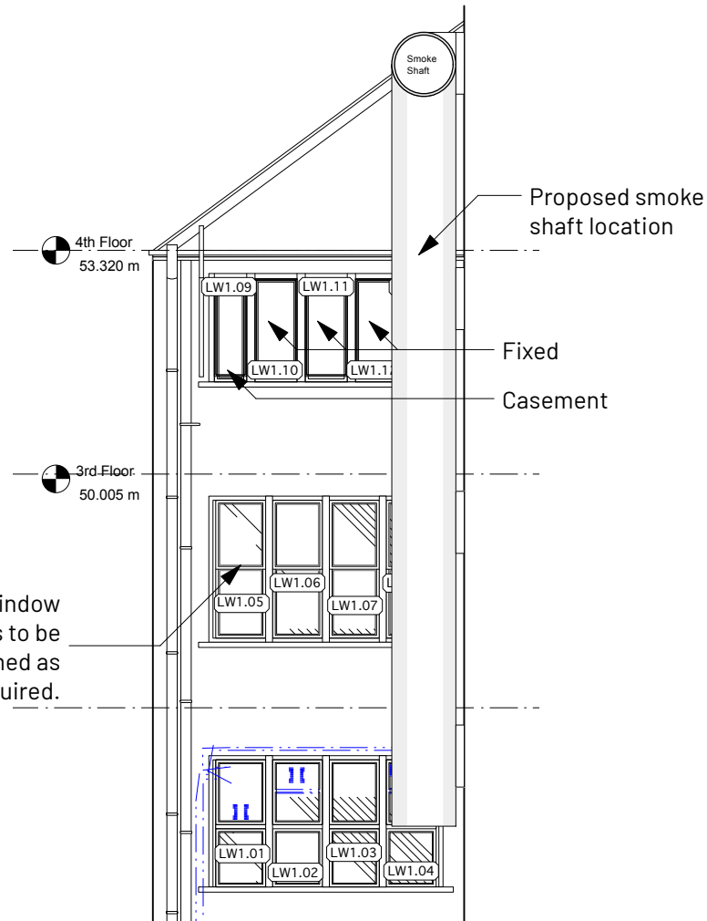
4 Section C-C Scale: 1:100
