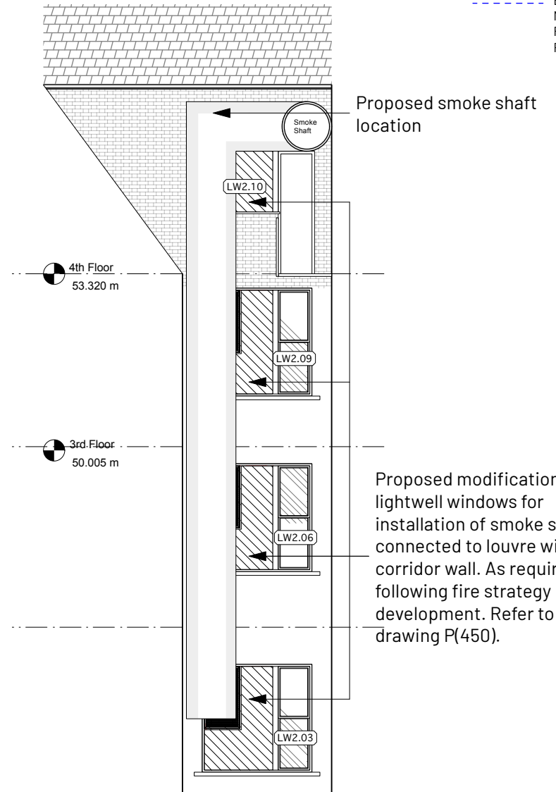
5 Section D-D Scale: 1:100
