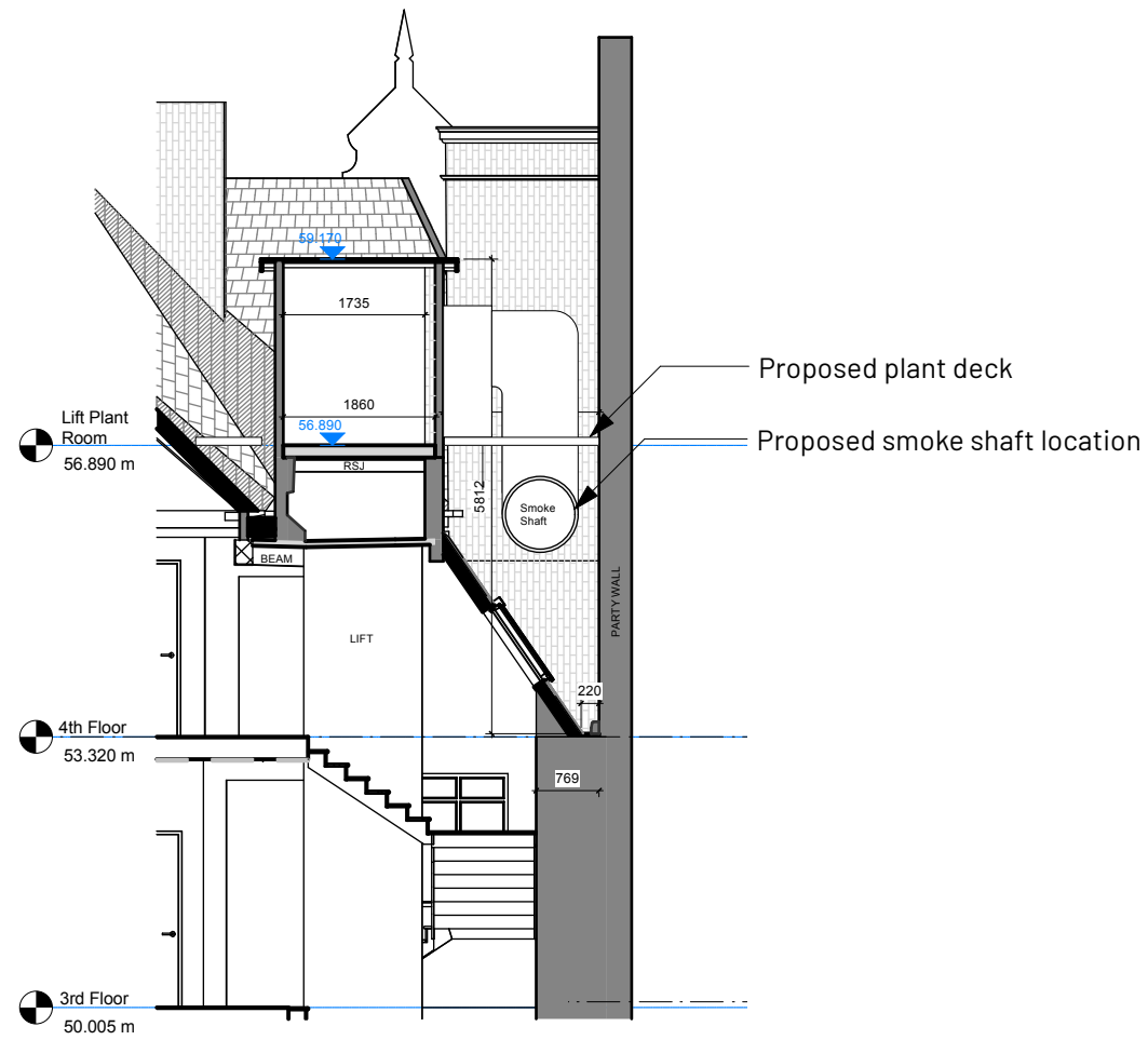
2 Section A-A Scale: 1:100
