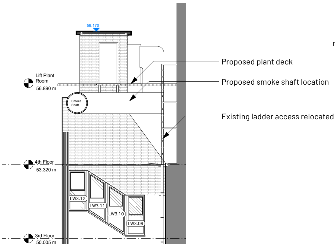
3 Section B-B Scale: 1:100
