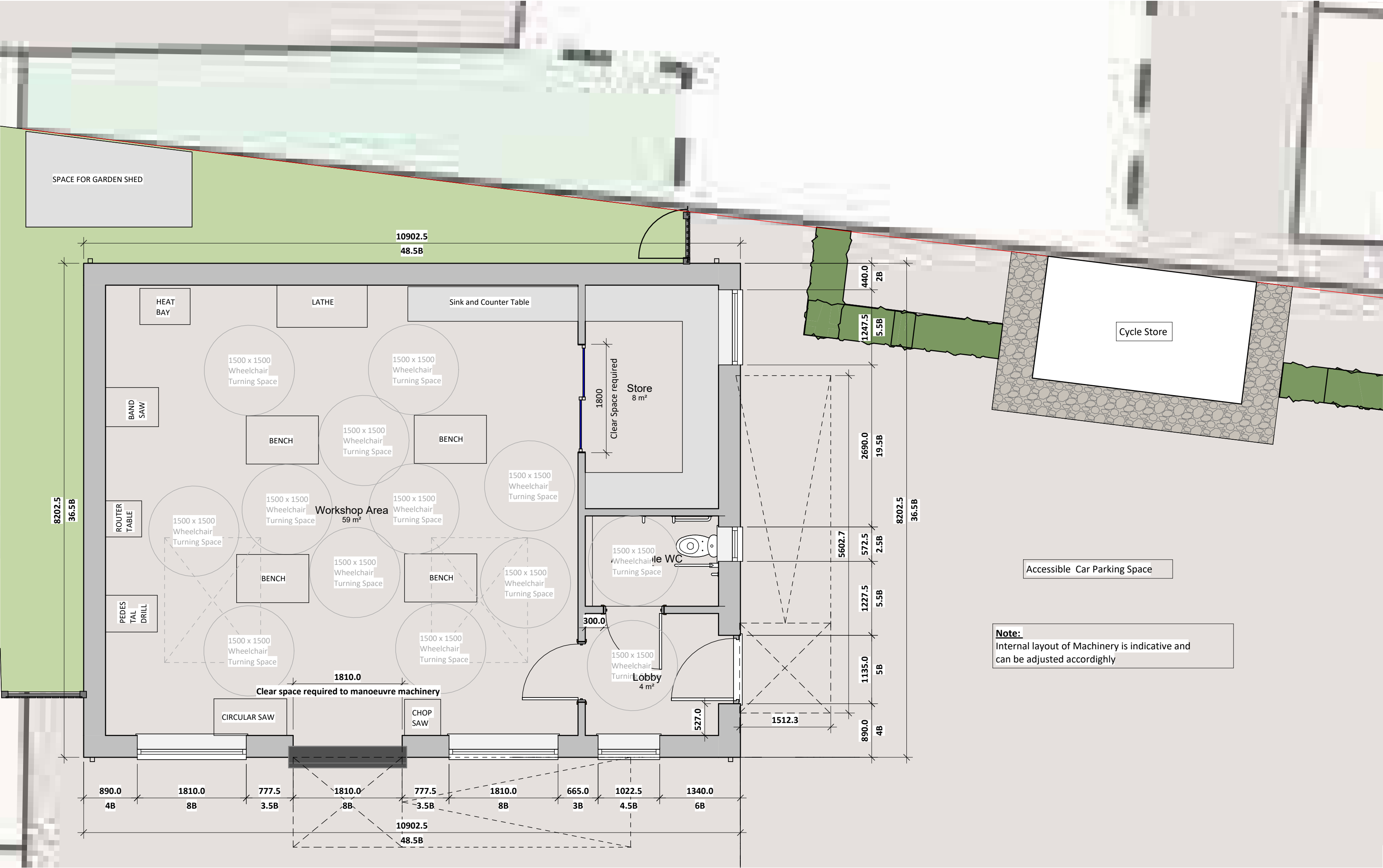
Workshop Plan 1 : 50
