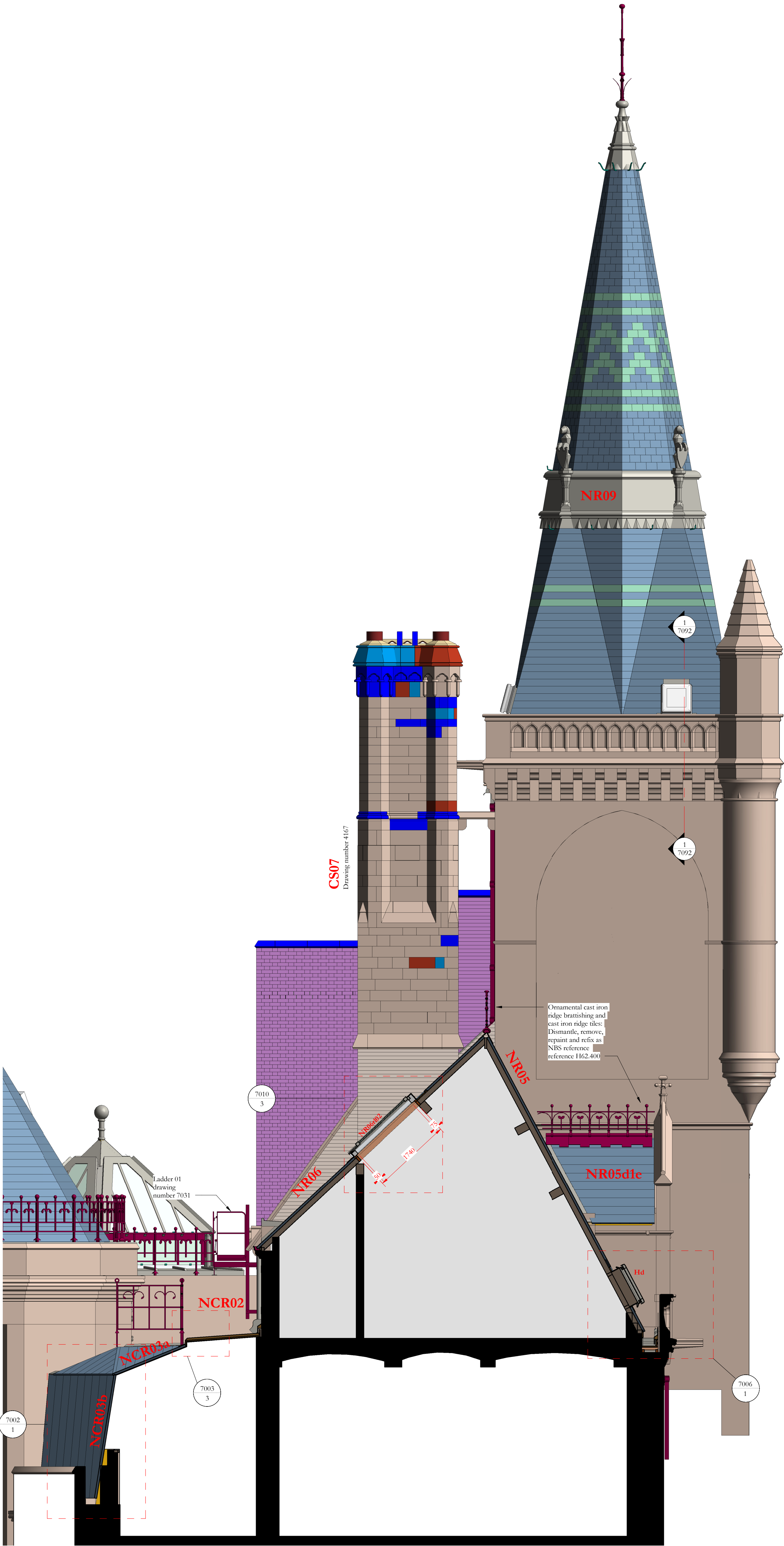
Section NN 1 : 50
