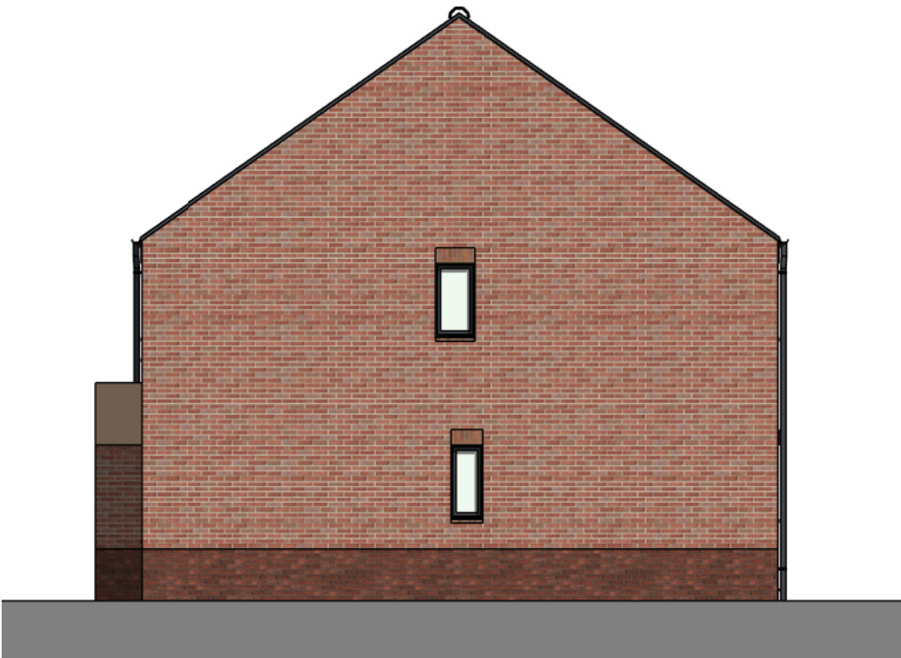
Right Elevation 1 : 100
