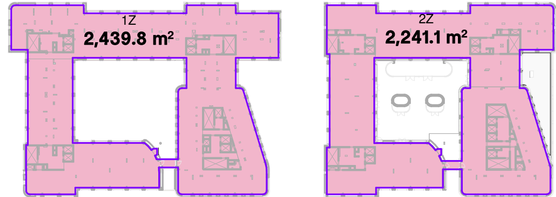
2 GIA - L01 1 : 1000
