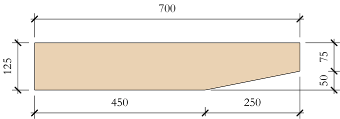
TcW_03 Elevation Top 1 : 10
