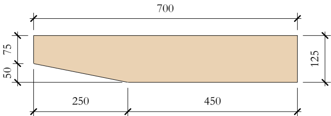
TcW_04 Elevation Top 1 : 10
