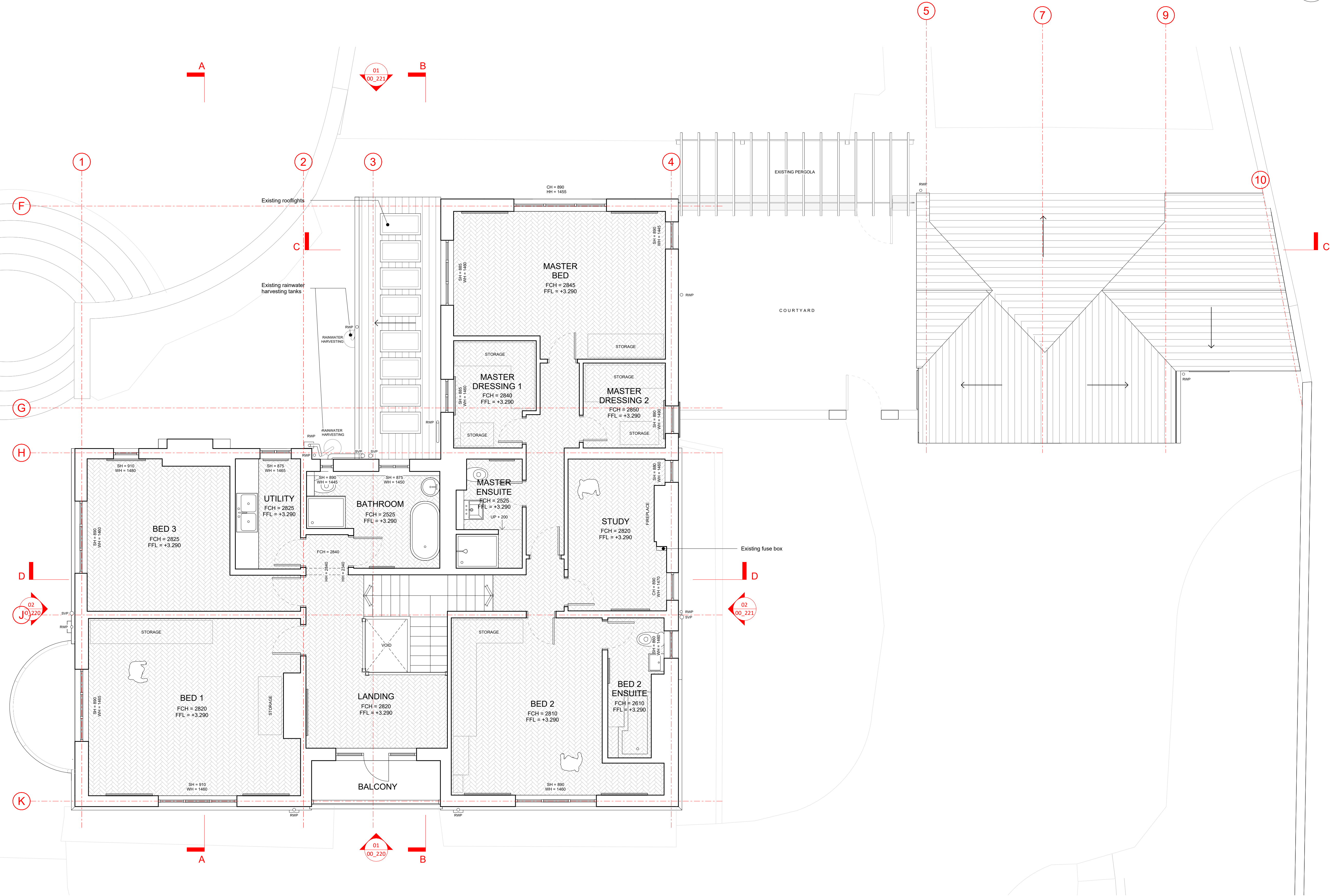
01 EXISTING L1 PLAN 1 : 50
