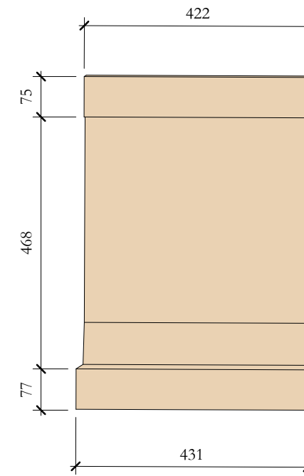
Elevation Top 1 : 10
