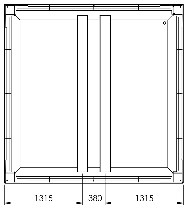
SECTION B-B SCALE 1 : 30
