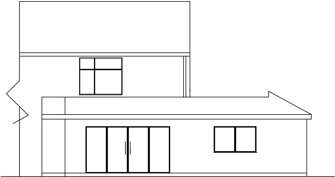
Elevation B
