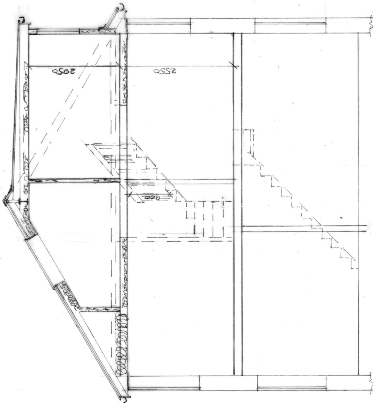
SECTION A-A
