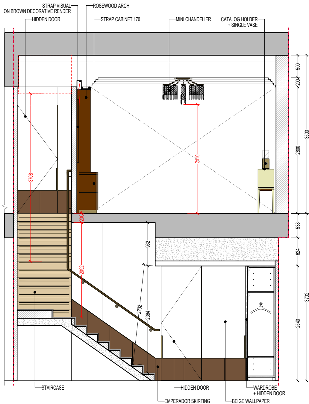
ELEVATION 6
