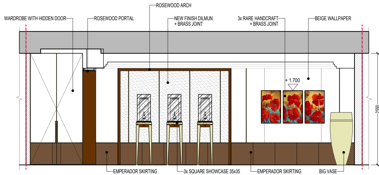
ELEVATION 9
