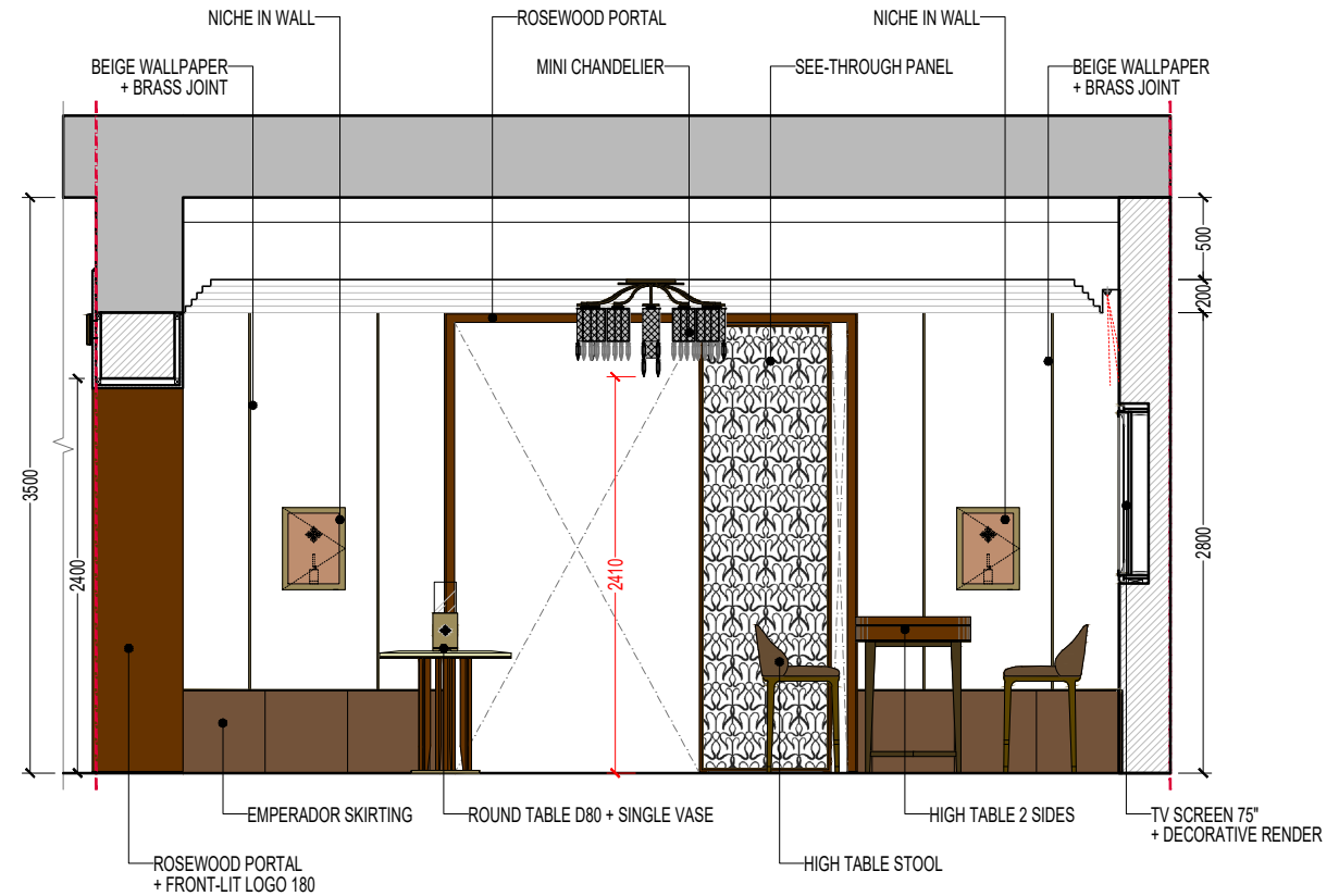
ELEVATION 4
