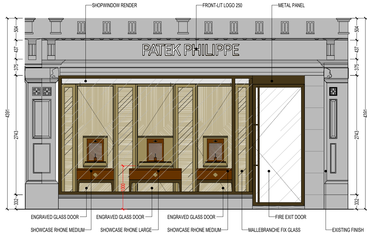
ELEVATION A
