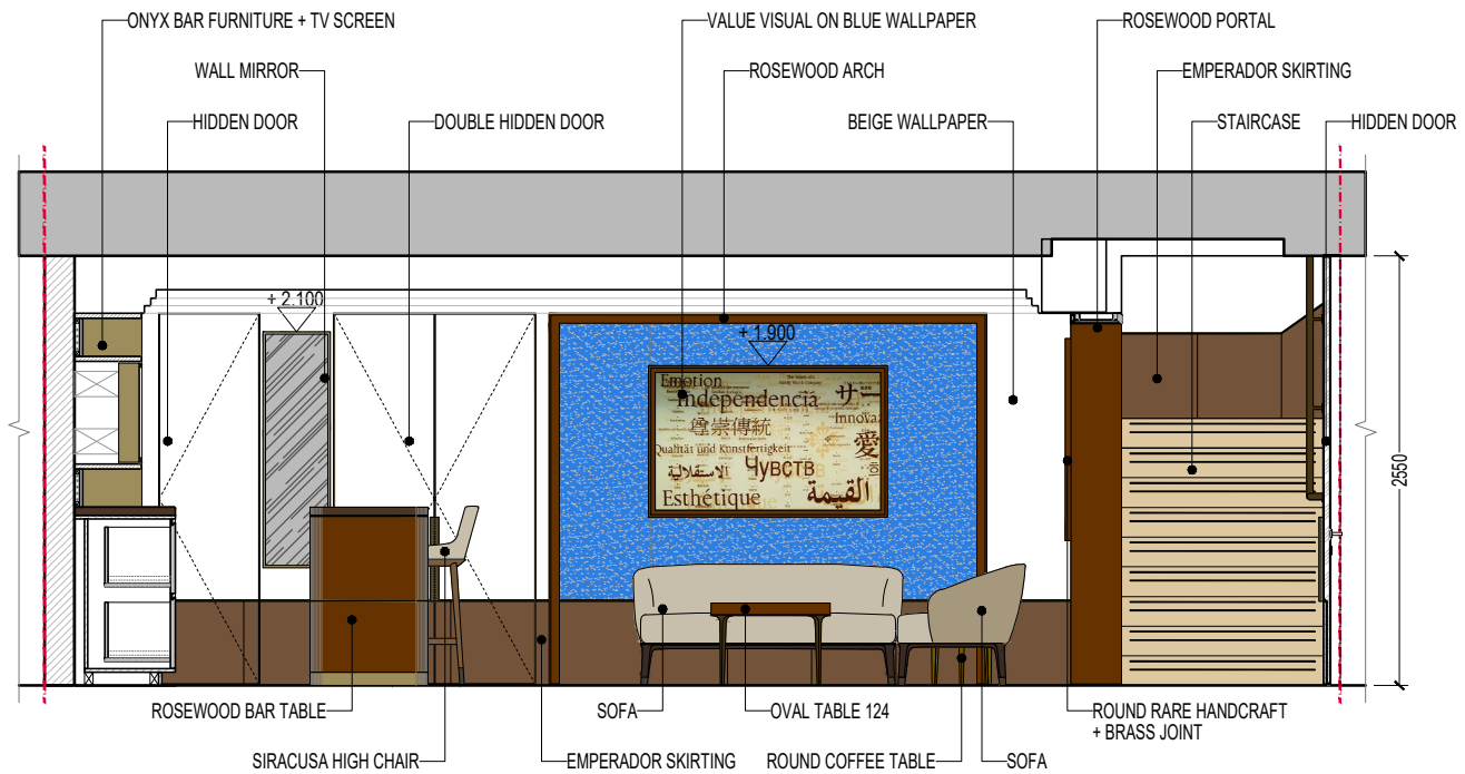
ELEVATION 11
