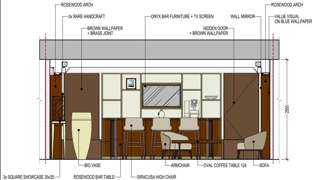
ELEVATION 10
