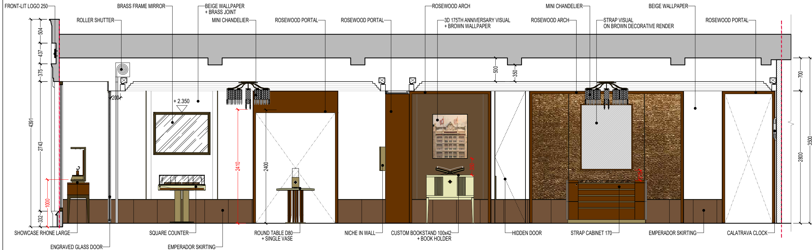
ELEVATION 2
