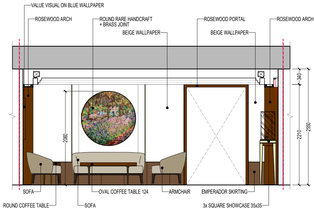
ELEVATION 8
