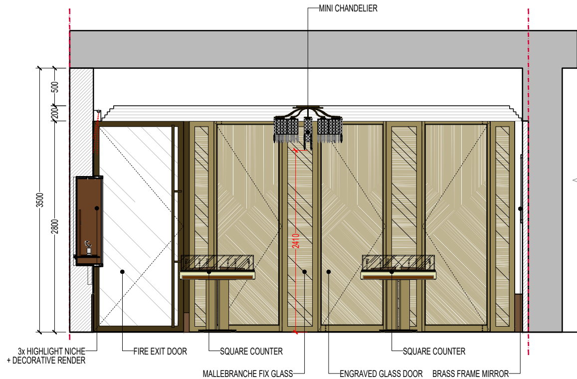
ELEVATION 1
