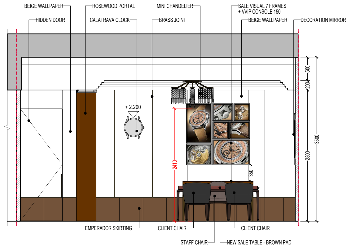
ELEVATION 7
