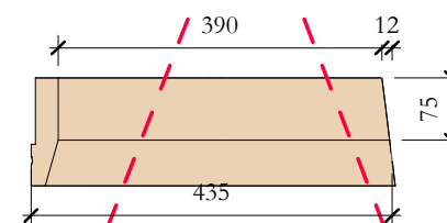
TcH_03 Elevation Top 1 : 10
