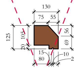
TcH_03 Cross Section 1 : 10
