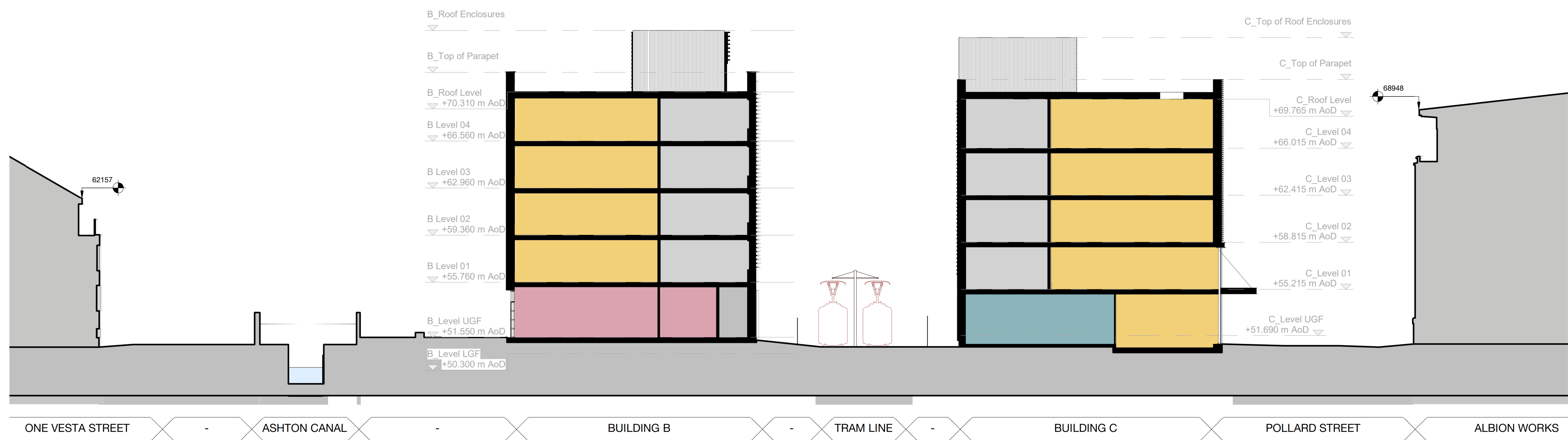
Site Section CC. 1 : 200
