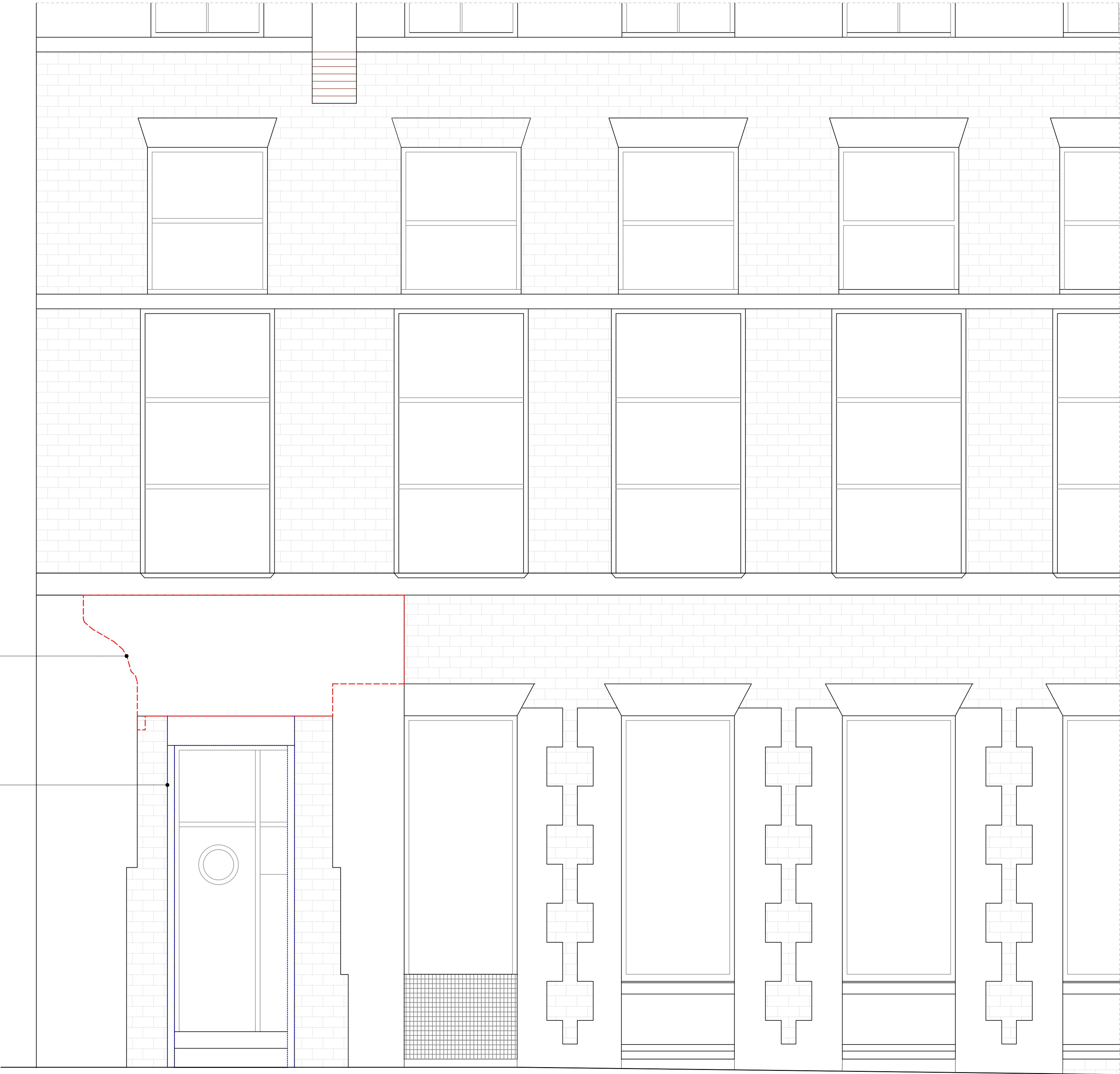
1 EXISTING ELEVATION Scale: 1:25
