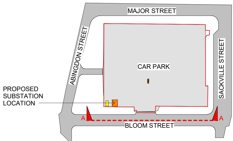
KEY PLAN 1 : 1000
