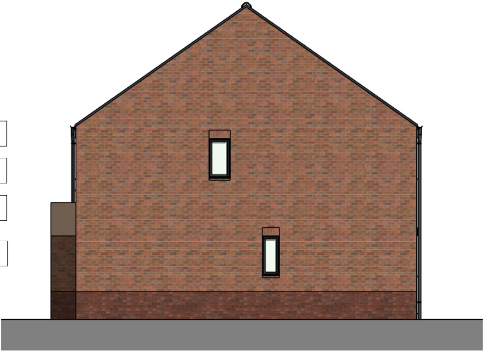
Right Elevation 1 : 100
