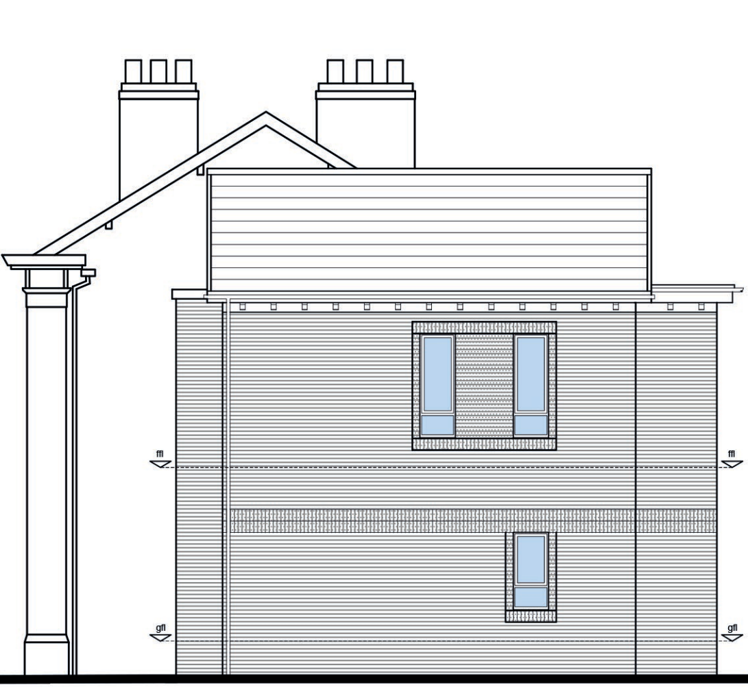
R.H Side Elevation Type E
