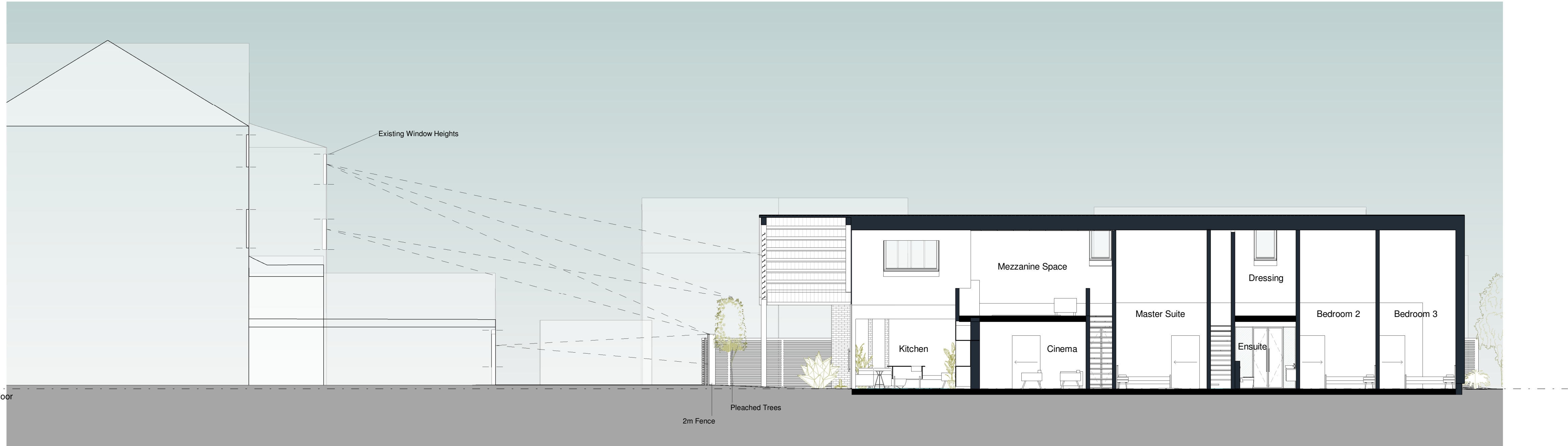
Section B-B 1 : 100
