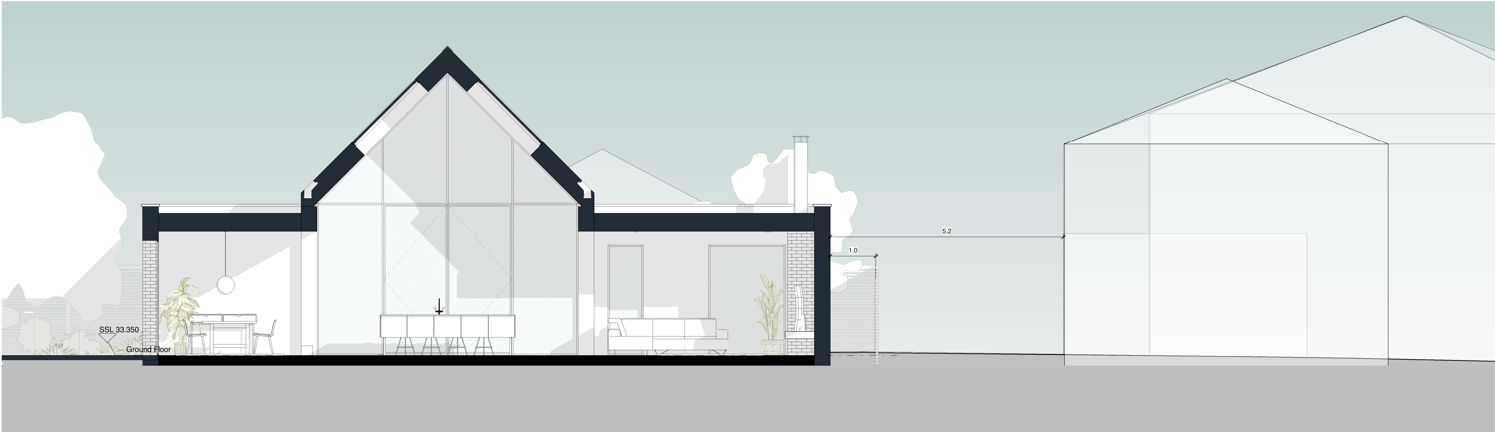
Section A-A 1 : 50
