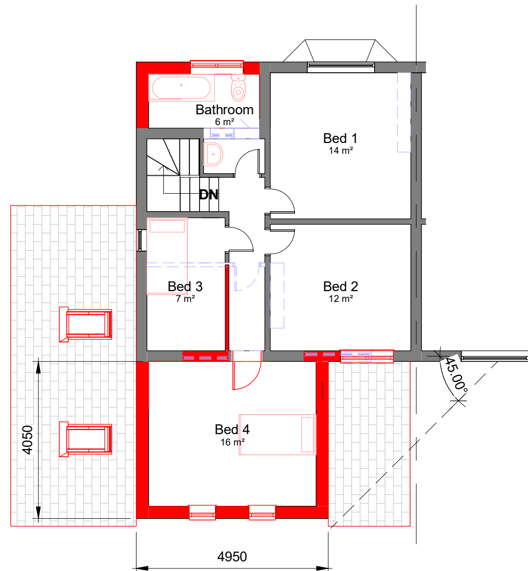
01-P-First Floor 1 : 100
