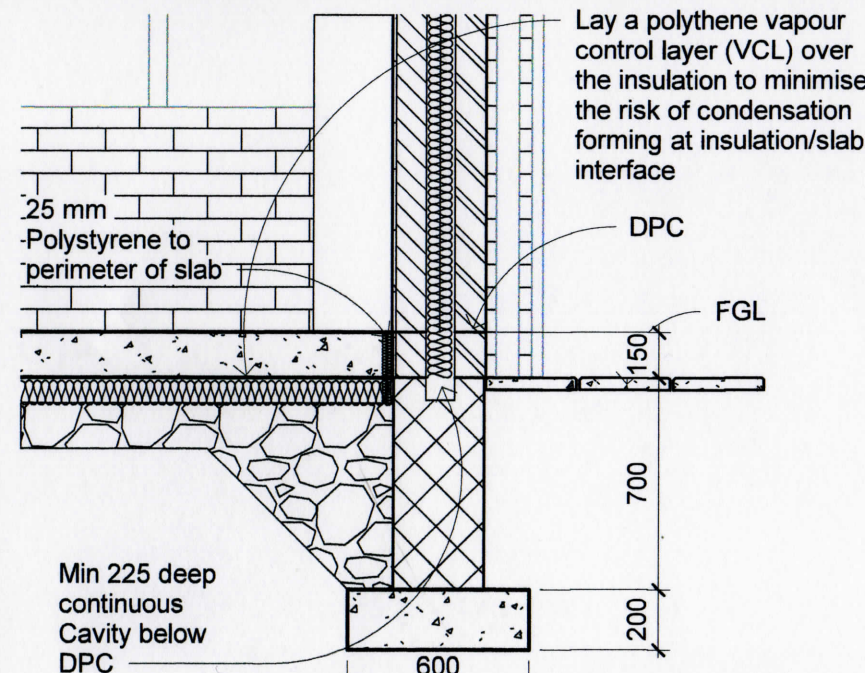
1 Section 1 - Callout 1 1 : 25
