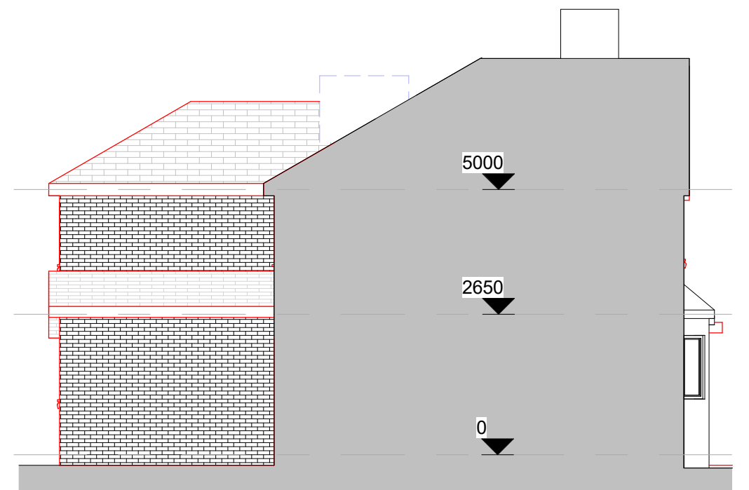
04-P-Elevation 1 : 100
