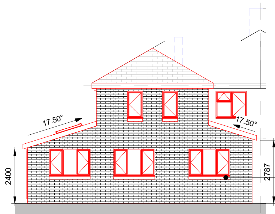
03-P-Elevation 1 : 100
